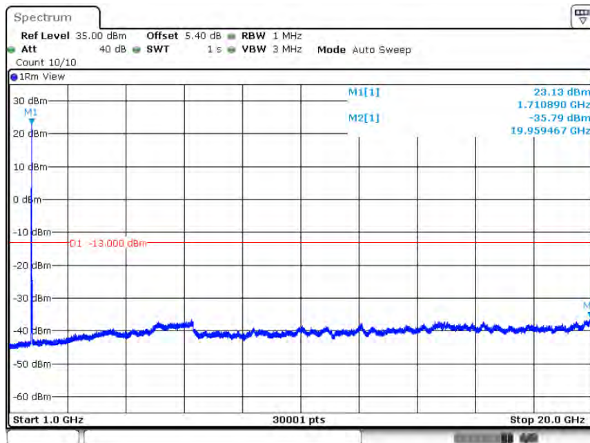
Band4-20MHz-QPSK-20050-1RB#0-Range2:1000~20000MHz
