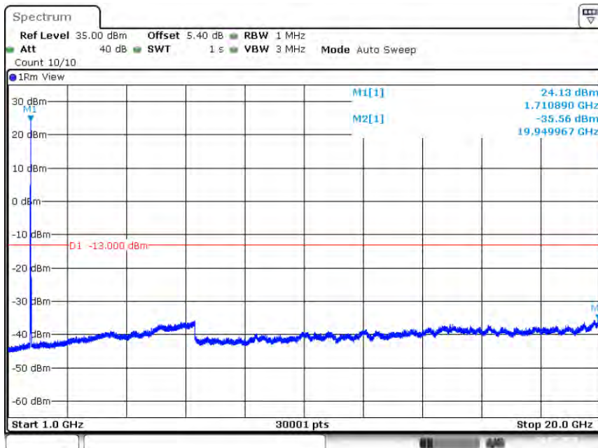
Band66-20MHz-QPSK-132072-1RB#0-Range2:1000~20000MHz
