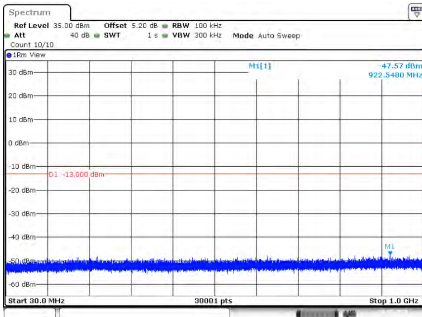
Band66-20MHz-QPSK-132072-1RB#0-Range1:30~1000MHz
