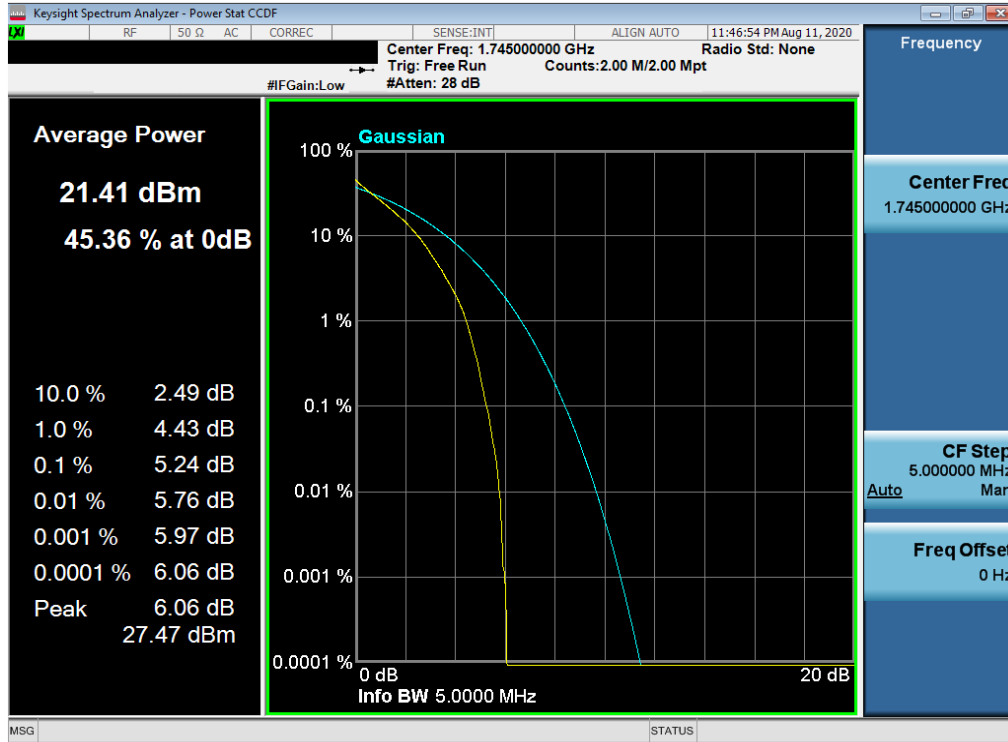
Plot 7-488. PAR Plot (LTE Band 66/4 - 5MHz QPSK - Full RB Configuration)
