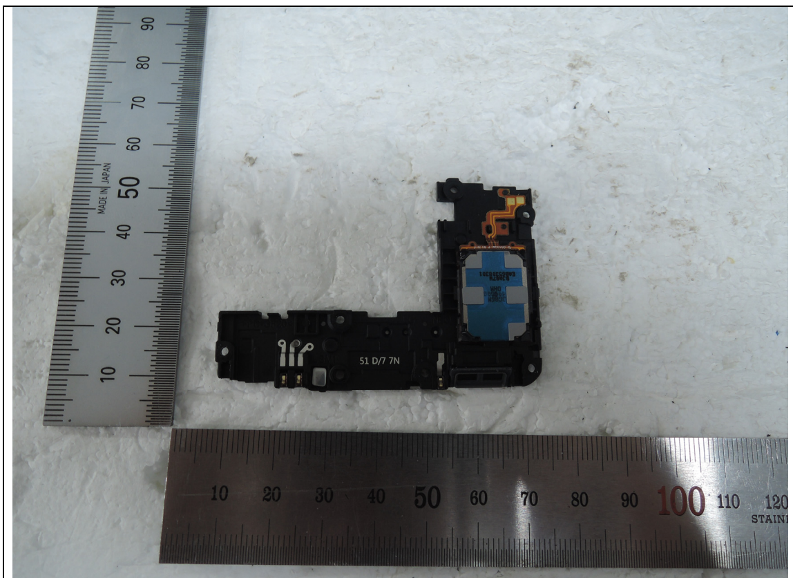
&lt;Antenna&gt;
