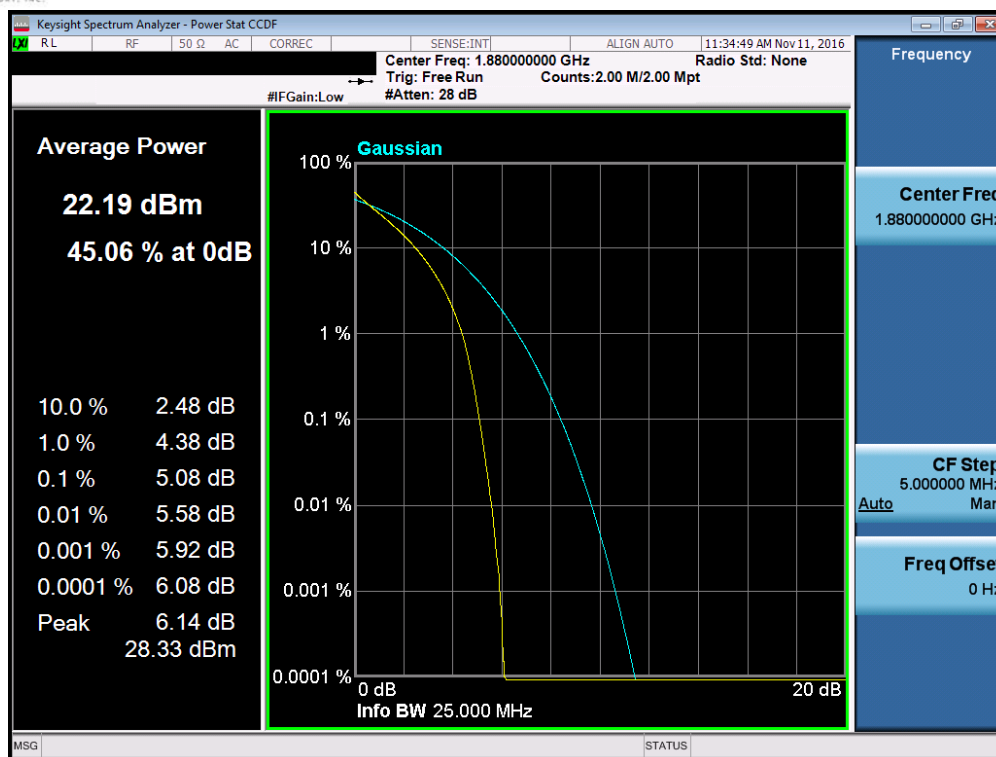
Plot 7-163. PAR Plot (Band 2 – 20.0MHz QPSK – RB Size 100)
