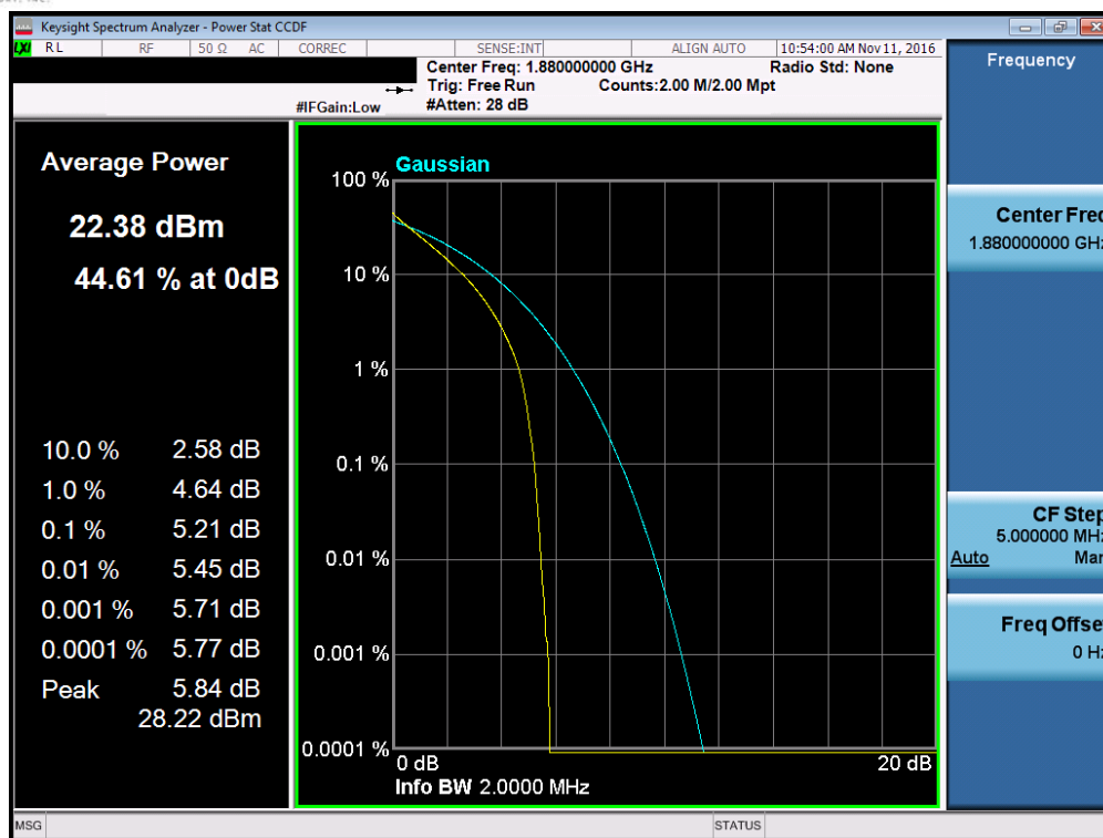
Plot 7-153. PAR Plot (Band 2 – 1.4MHz QPSK – RB Size 6)
