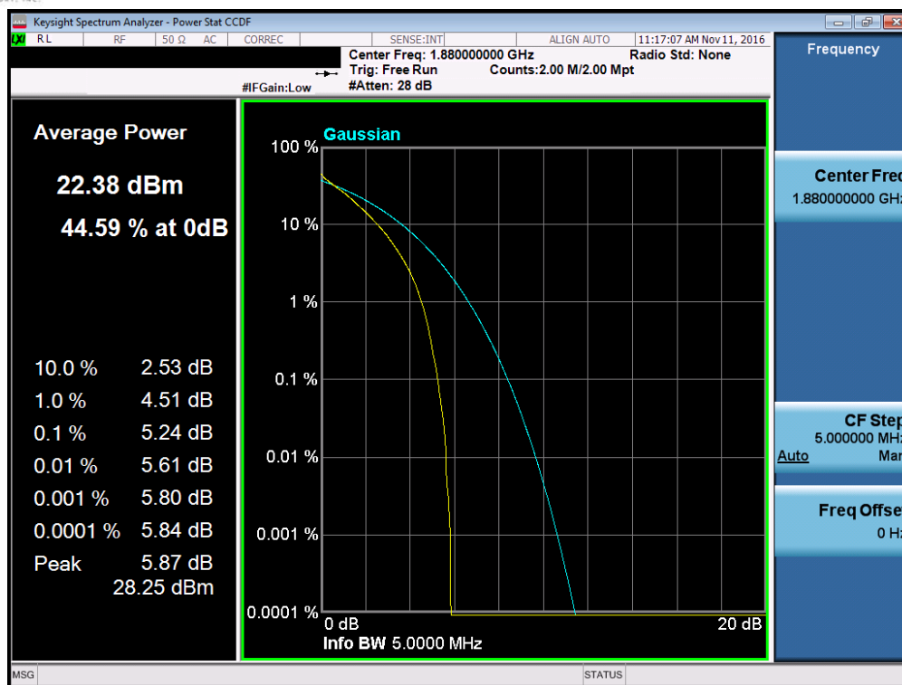
Plot 7-157. PAR Plot (Band 2 – 5.0MHz QPSK – RB Size 25)
