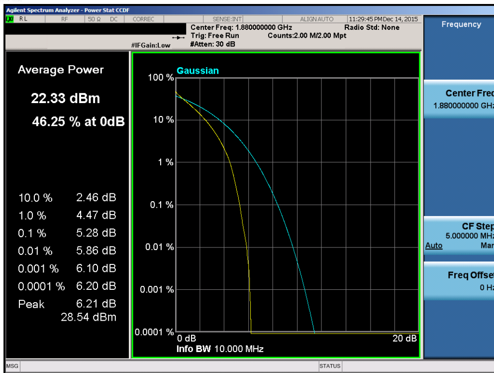
Plot 7-118. PAR Plot (Band 2 – 10.0MHz QPSK – RB Size 50)
