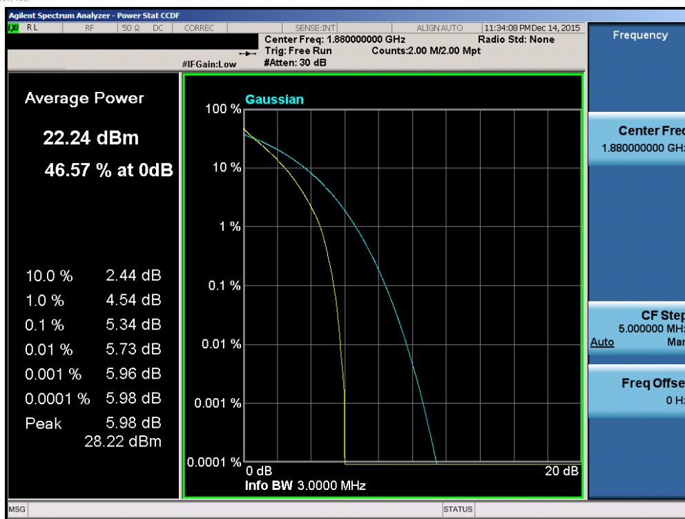
Plot 7-114. PAR Plot (Band 2 – 3.0MHz QPSK – RB Size 15)
