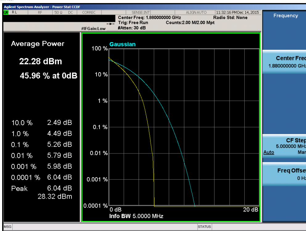
Plot 7-116. PAR Plot (Band 2 – 5.0MHz QPSK – RB Size 25)
