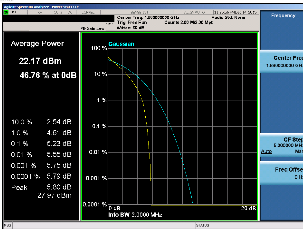
Plot 7-112. PAR Plot (Band 2 – 1.4MHz QPSK – RB Size 6)
