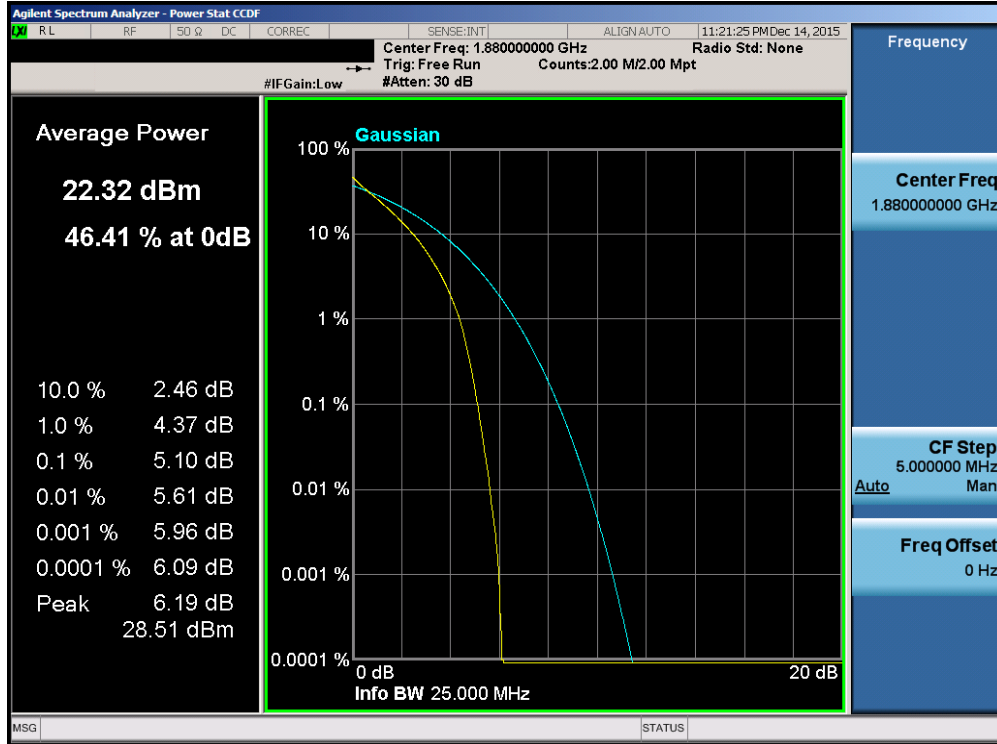
Plot 7-122. PAR Plot (Band 2 – 20.0MHz QPSK – RB Size 100)
