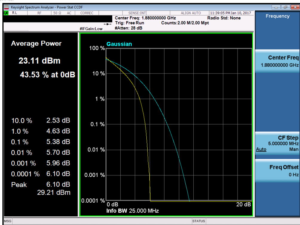
Plot 7-114. PAR Plot (Band 2 – 15.0MHz QPSK – RB Size 75)
