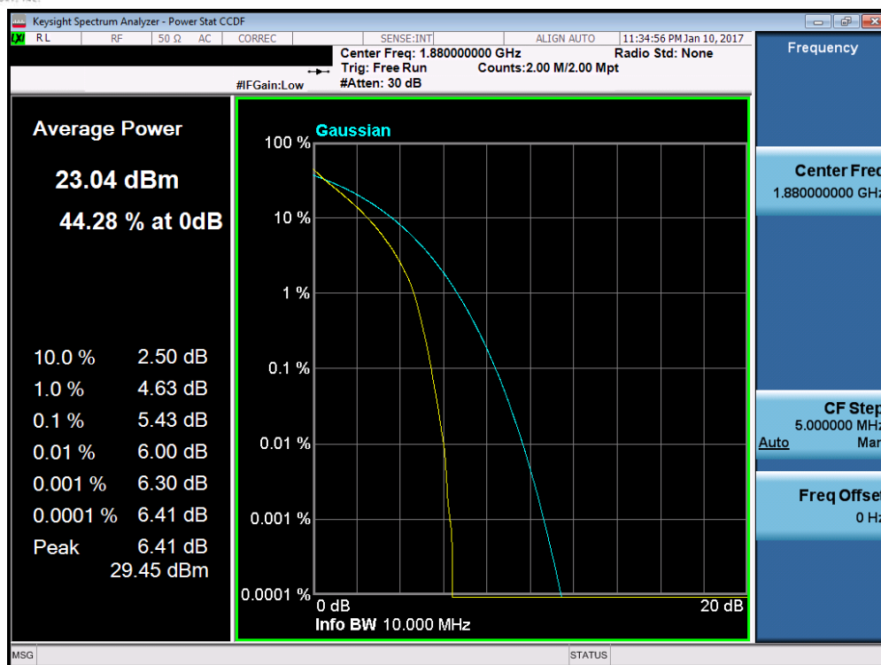
Plot 7-112. PAR Plot (Band 2 – 10.0MHz QPSK – RB Size 50)
