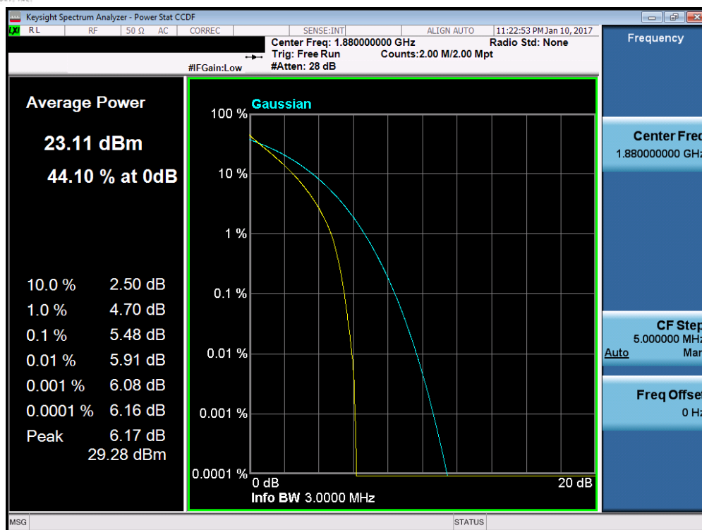
Plot 7-108. PAR Plot (Band 2 – 3.0MHz QPSK – RB Size 15)
