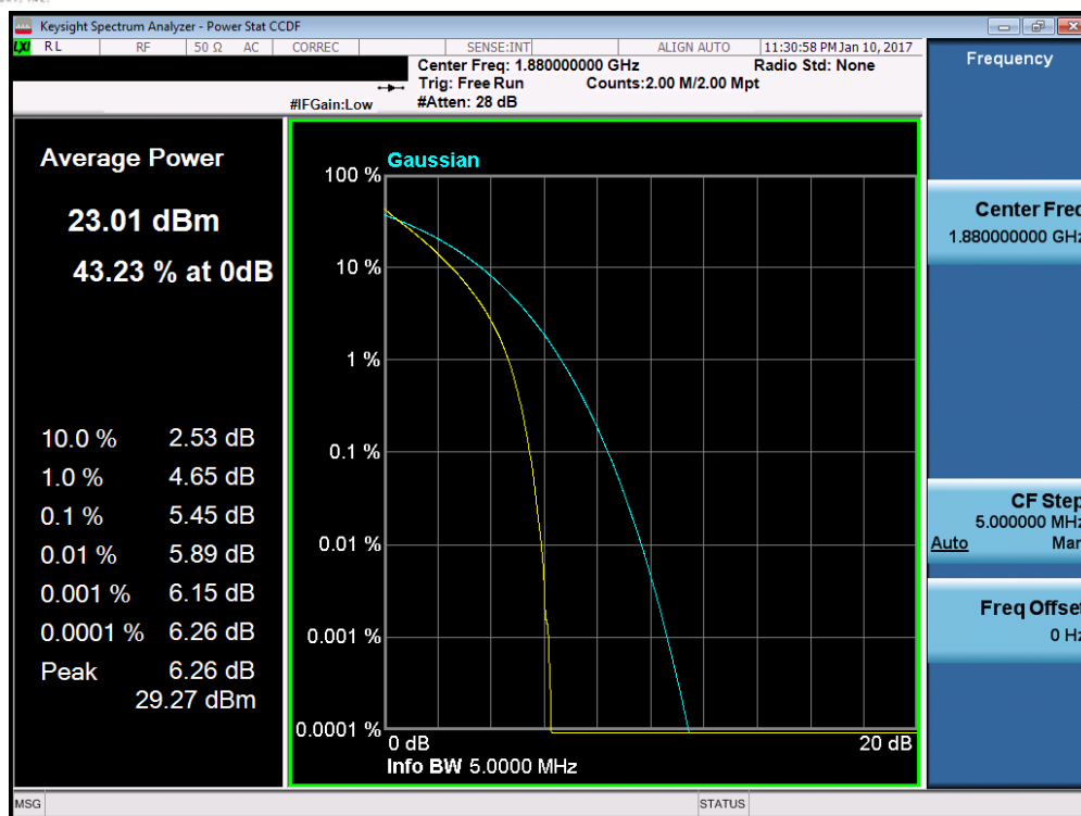
Plot 7-110. PAR Plot (Band 2 – 5.0MHz QPSK – RB Size 25)
