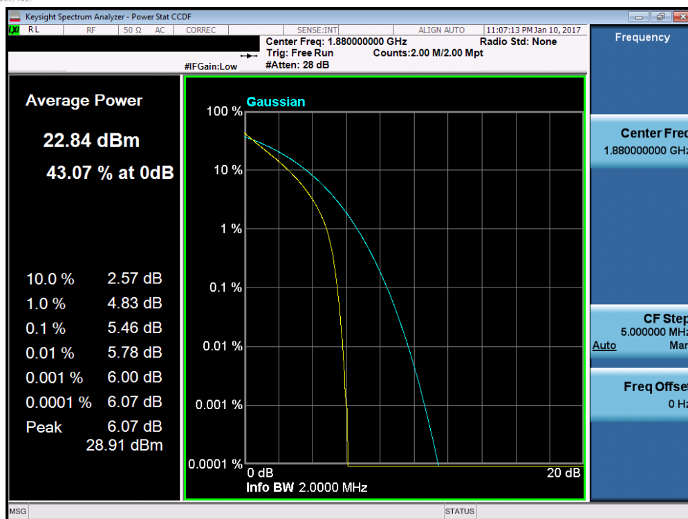
Plot 7-106. PAR Plot (Band 2 – 1.4MHz QPSK – RB Size 6)
