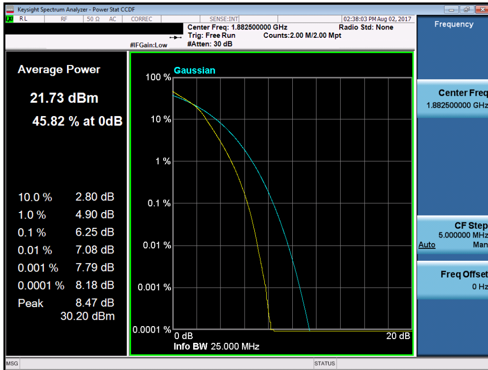
Plot 7-193. PAR Plot (Band 2/25 – 20.0MHz 16-QAM – RB Size 100)
