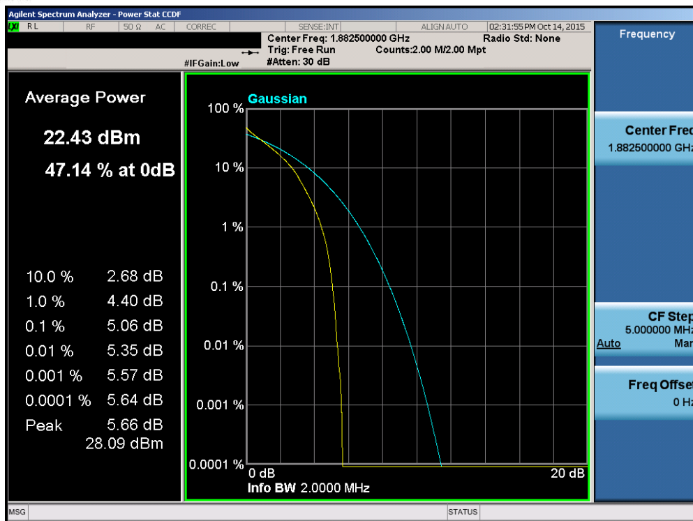
Plot 7-133. PAR Plot (Band 25 – 1.4MHz QPSK – RB Size 6)
