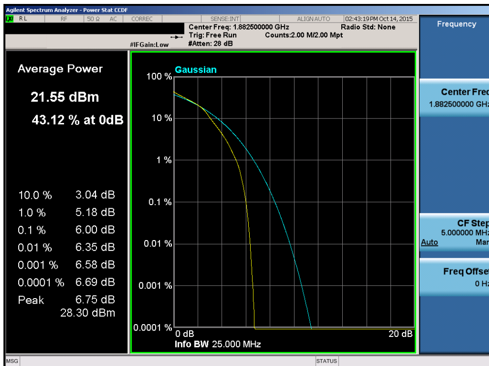
Plot 7-142. PAR Plot (Band 25 – 15.0MHz 16-QAM – RB Size 75)
