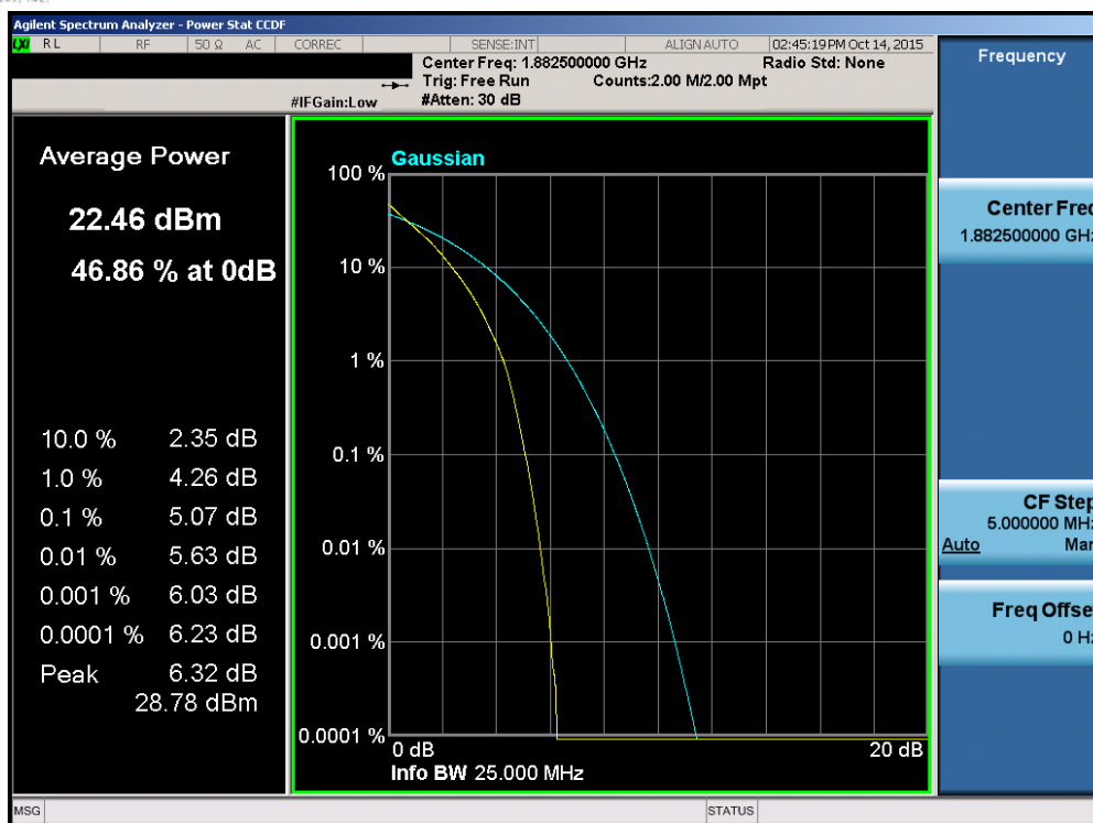
Plot 7-143. PAR Plot (Band 25 – 20.0MHz QPSK – RB Size 100)
