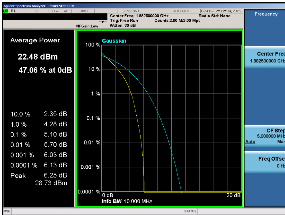
Plot 7-139. PAR Plot (Band 25 – 10.0MHz QPSK – RB Size 50)
