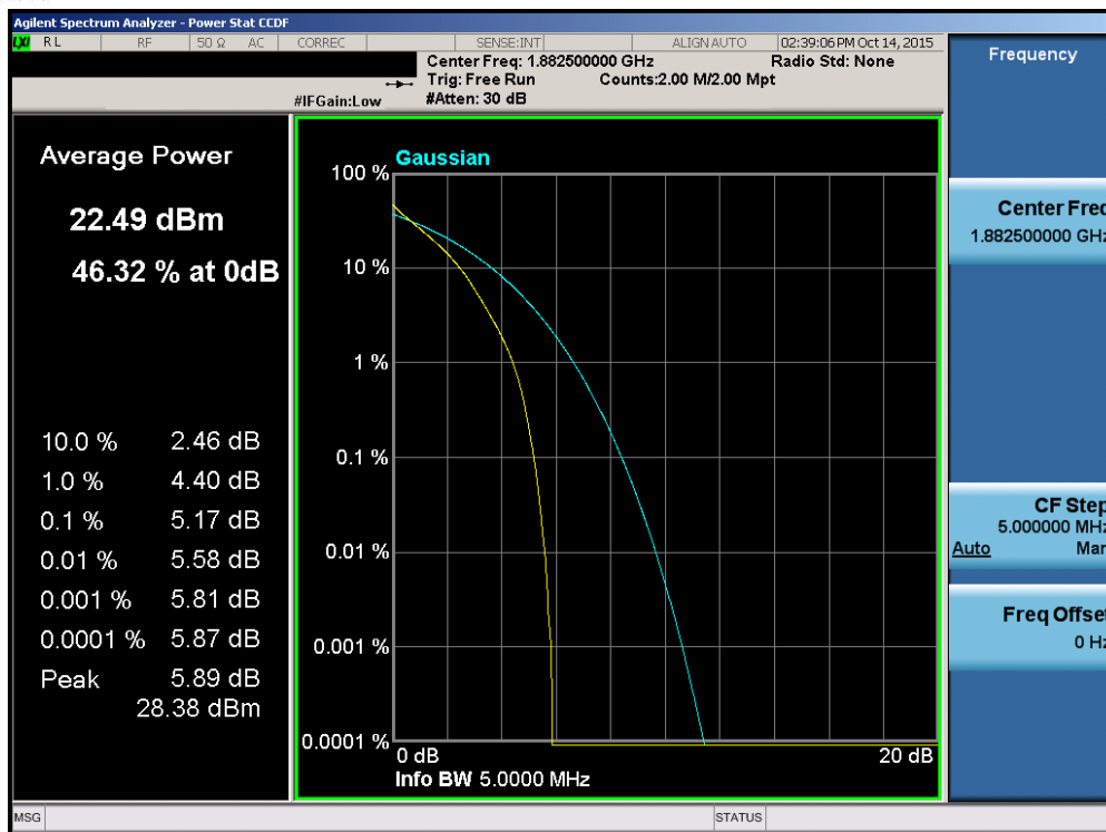
Plot 7-137. PAR Plot (Band 25 – 5.0MHz QPSK – RB Size 25)
