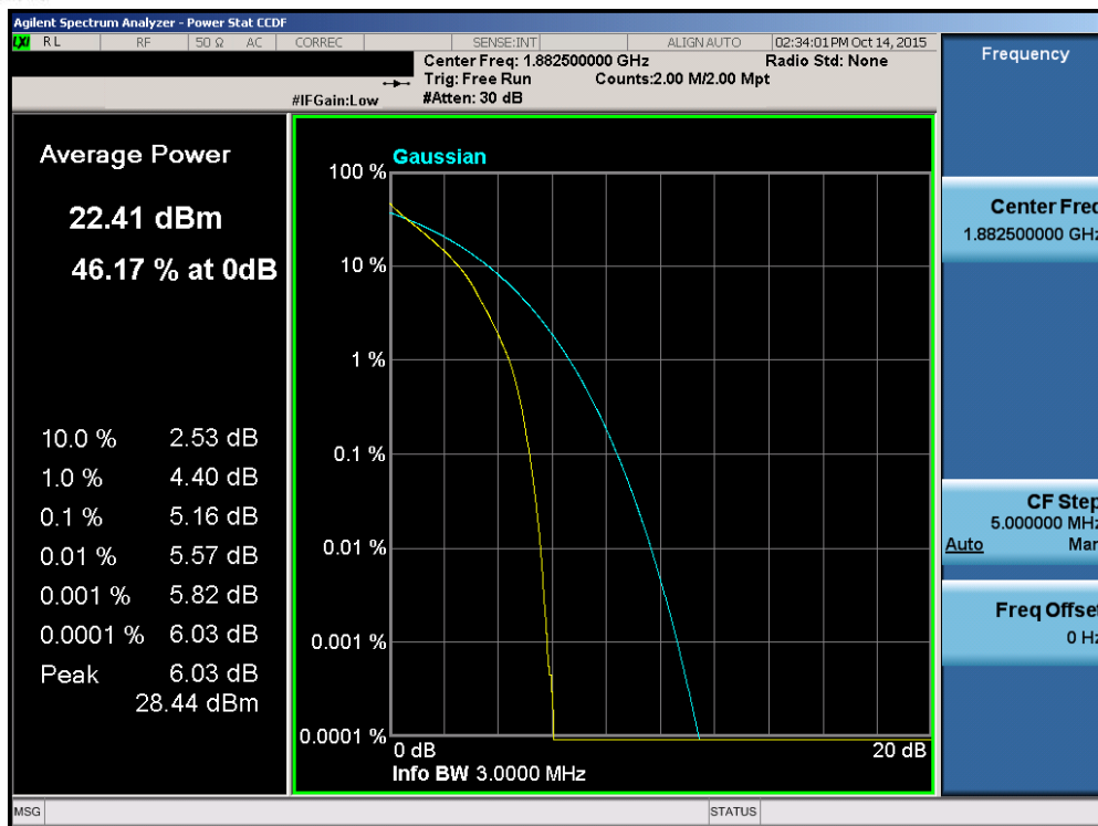
Plot 7-135. PAR Plot (Band 25 – 3.0MHz QPSK – RB Size 15)
