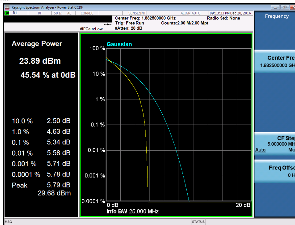
Plot 7-229. PAR Plot (Band 25/2 – 15.0MHz QPSK – RB Size 75)
