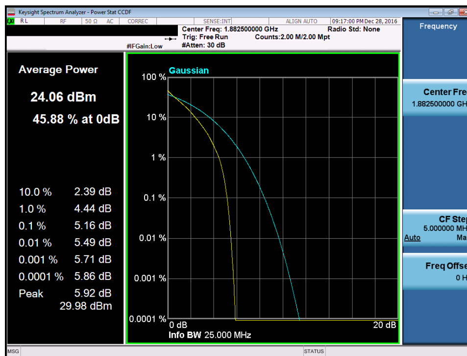
Plot 7-232. PAR Plot (Band 25/2 - 20.0MHz QPSK - RB Size 100)
