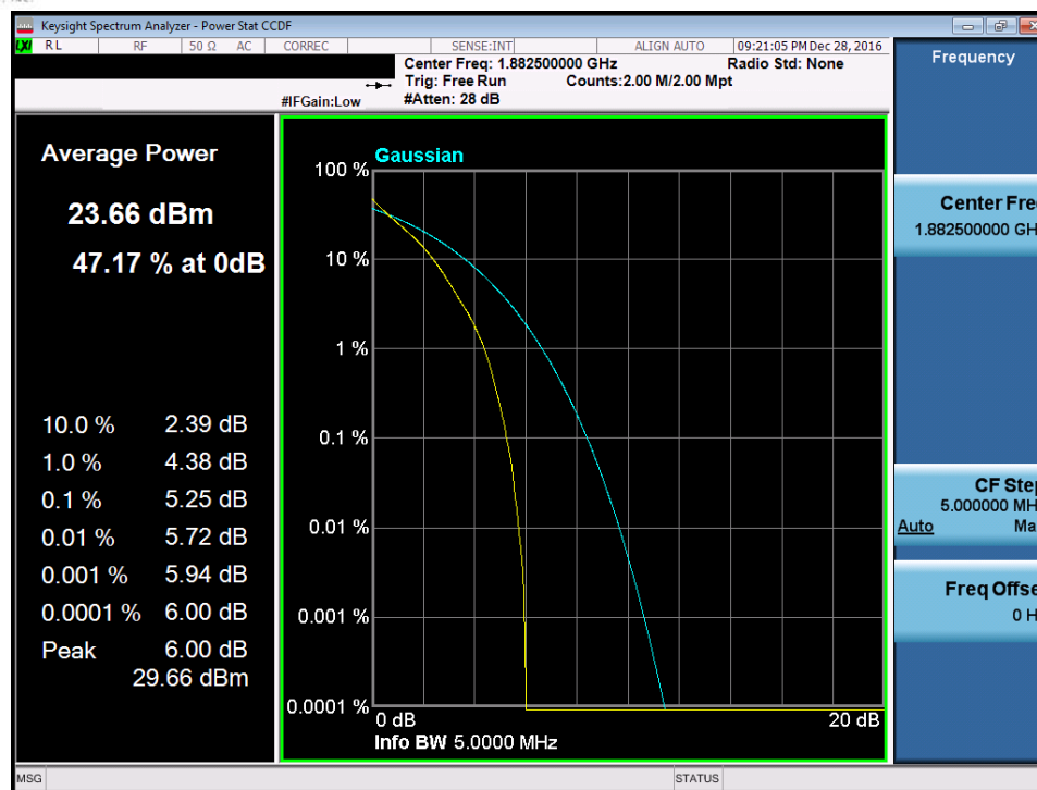
Plot 7-223. PAR Plot (Band 25/2 – 5.0MHz QPSK – RB Size 25)
