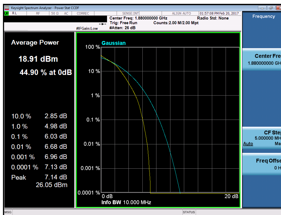
Plot 7-228. PAR Plot (Band 25/2 – 10.0MHz 64-QAM – RB Size 50)
