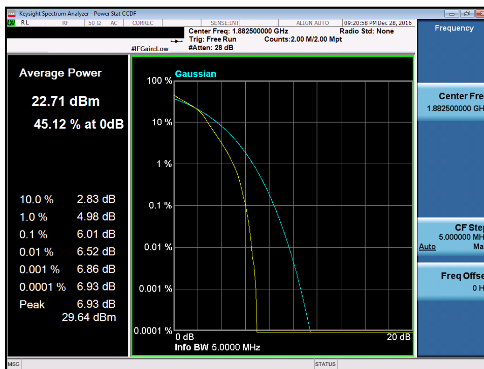
Plot 7-224. PAR Plot (Band 25/2 – 5.0MHz 16-QAM – RB Size 25)
