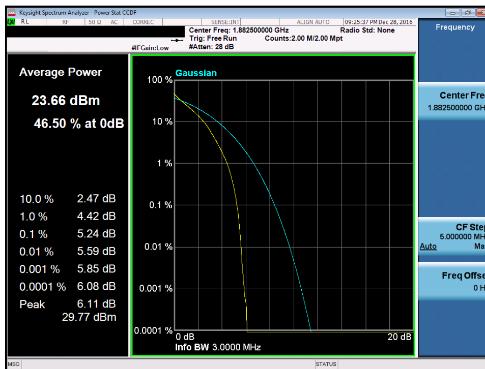
Plot 7-220. PAR Plot (Band 25/2 – 3.0MHz QPSK – RB Size 15)
