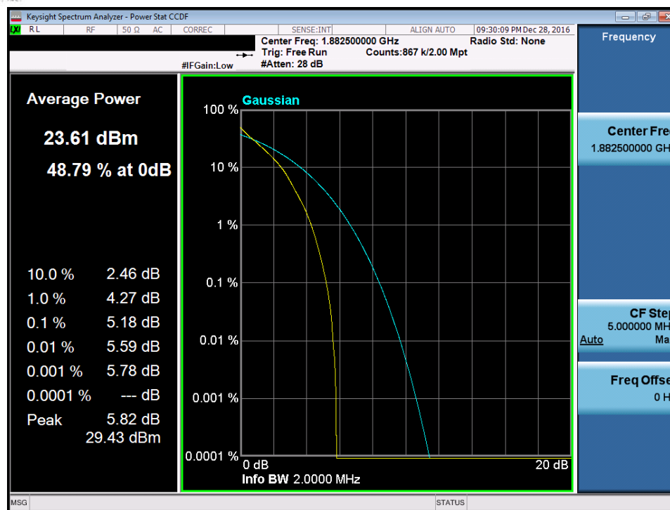
Plot 7-217. PAR Plot (Band 25/2 – 1.4MHz QPSK – RB Size 6)
