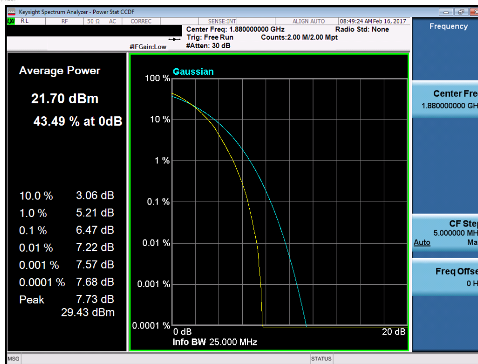
Plot 7-231. PAR Plot (Band 25/2 - 15.0MHz 64-QAM - RB Size 75)
