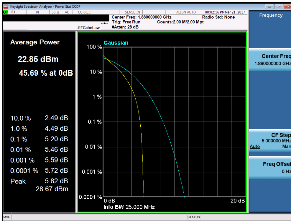
Plot 7-149. PAR Plot (Band 2 – 15.0MHz QPSK – RB Size 75)
