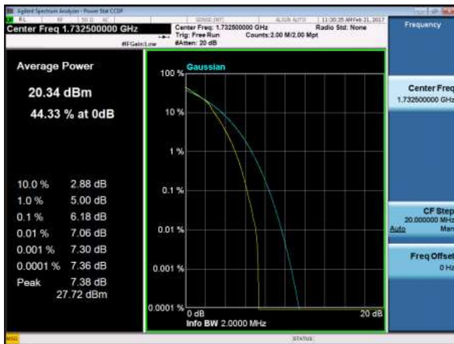
BAND 4. PAR Plot (1.4M BW_Ch.20175_16QAM_RB6_0)
