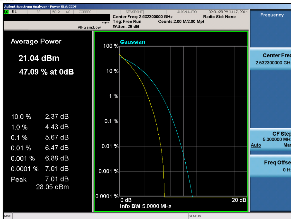
Plot 6-112. PAR Plot (Band 7 – 5.0MHz QPSK – RB Size 25)
