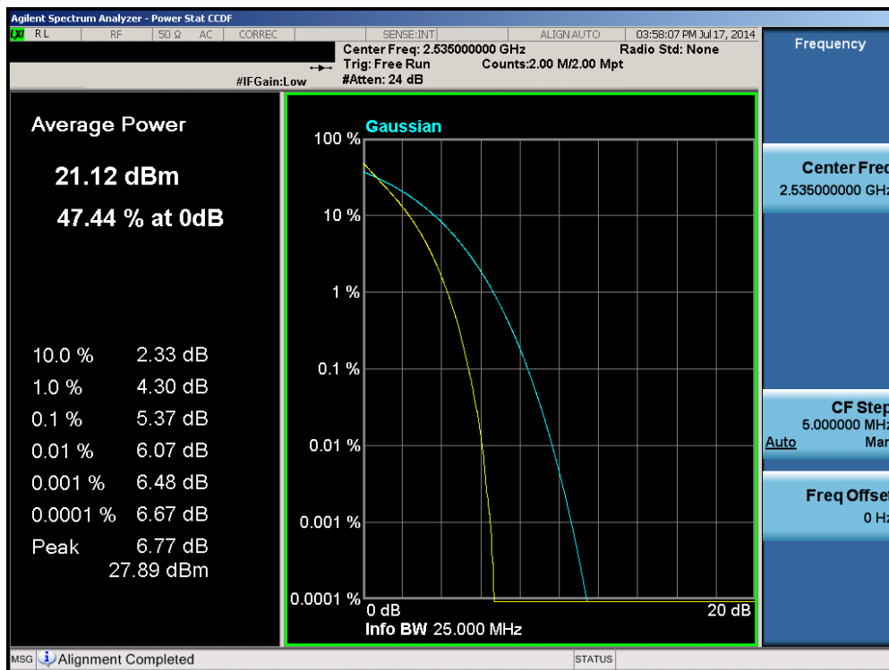
Plot 6-118. PAR Plot (Band 7 – 20.0MHz QPSK – RB Size 100)
