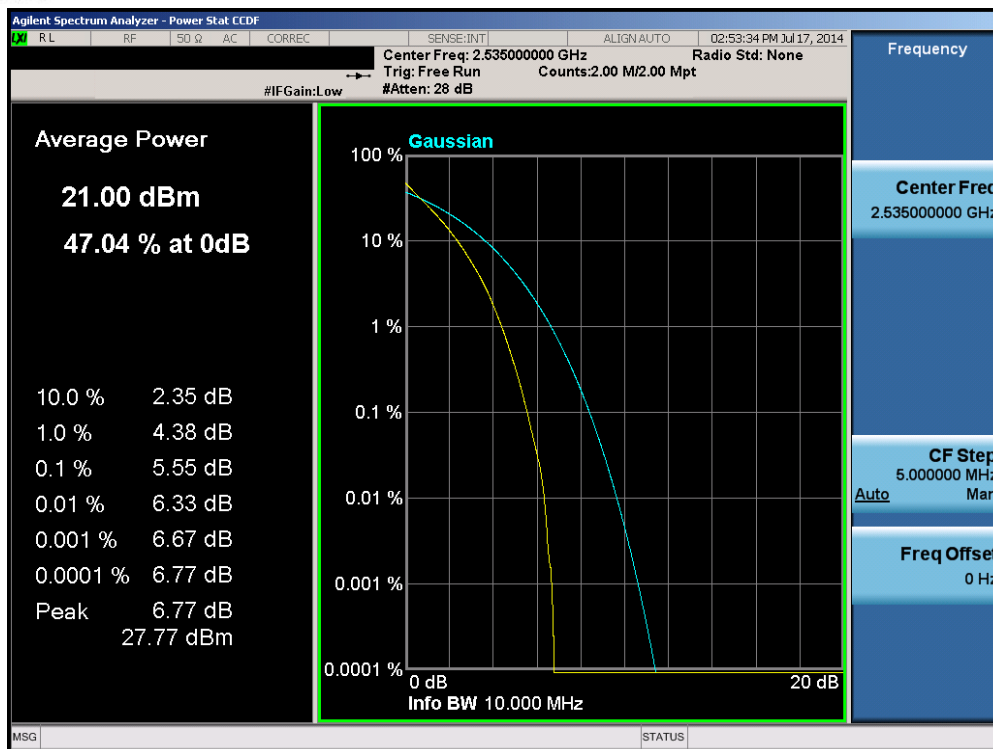
Plot 6-114. PAR Plot (Band 7 – 10.0MHz QPSK – RB Size 50)
