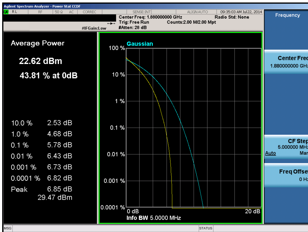
Plot 6-104. PAR Plot (Band 2 – 5.0MHz QPSK – RB Size 25)
