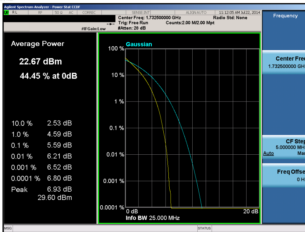
Plot 6-126. PAR Plot (Band 4 – 20.0MHz – QPSK – RB Size 100)
