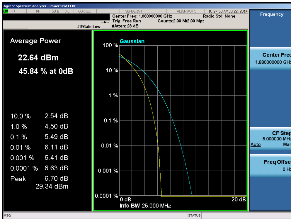
Plot 6-110. PAR Plot (Band 2 – 20.0MHz QPSK – RB Size 100)
