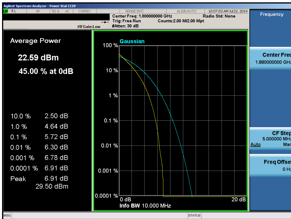
Plot 6-106. PAR Plot (Band 2 – 10.0MHz QPSK – RB Size 50)
