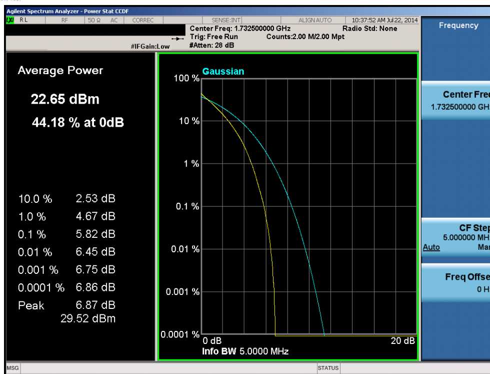
Plot 6-120. PAR Plot (Band 4 – 5.0MHz QPSK – RB Size 25)
