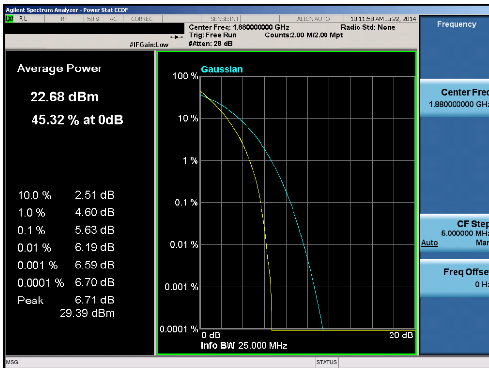
Plot 6-108. PAR Plot (Band 2 – 15.0MHz QPSK – RB Size 75)
