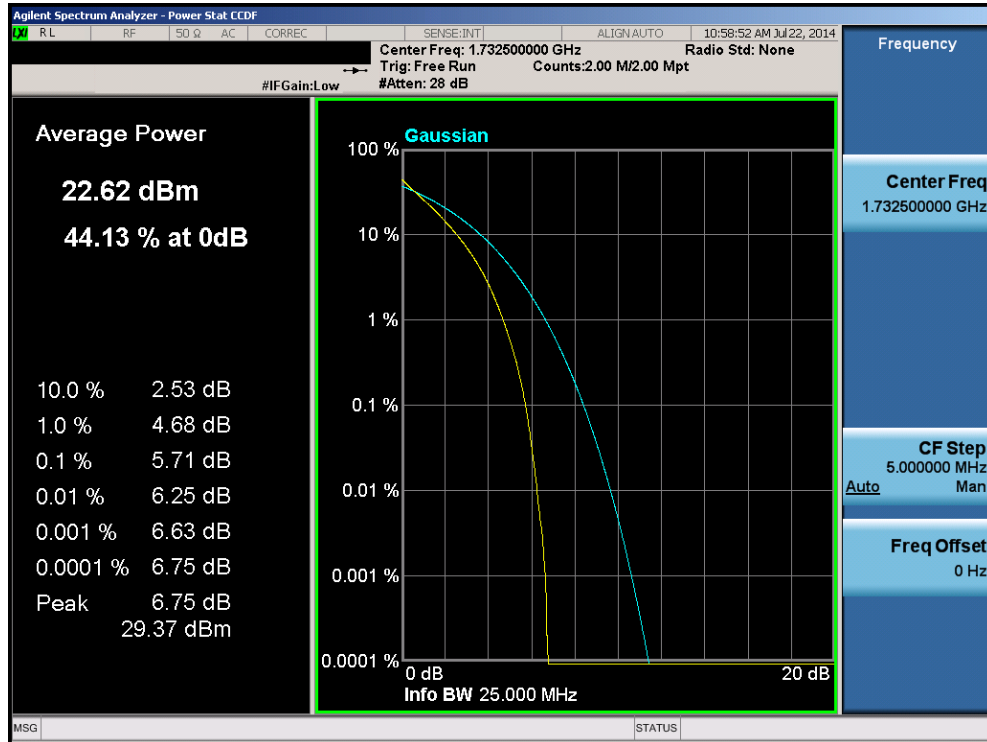
Plot 6-124. PAR Plot (Band 4 – 15.0MHz – QPSK – RB Size 75)
