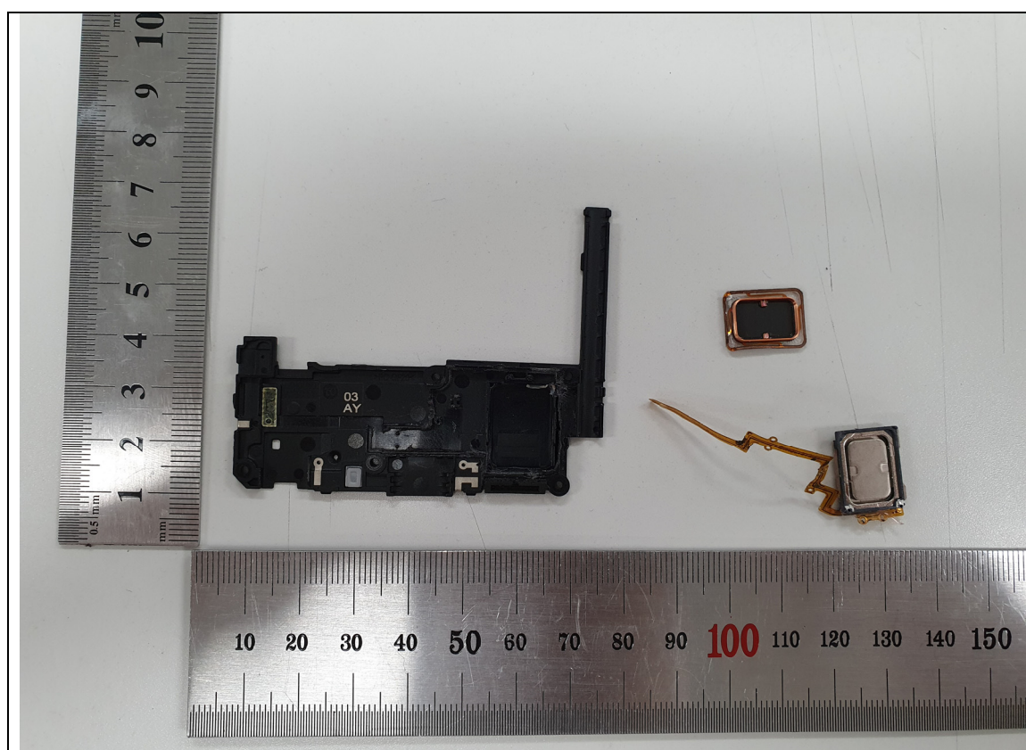
&lt;Antenna&gt;
