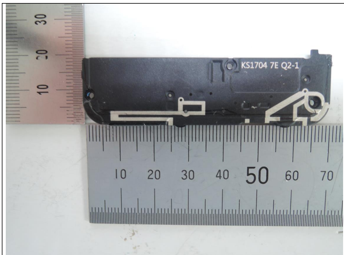
&lt;Antenna&gt;
