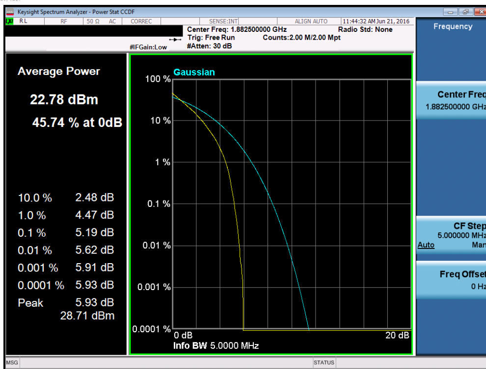
Plot 7-161. PAR Plot (Band 2/25 – 5.0MHz QPSK – RB Size 25)
