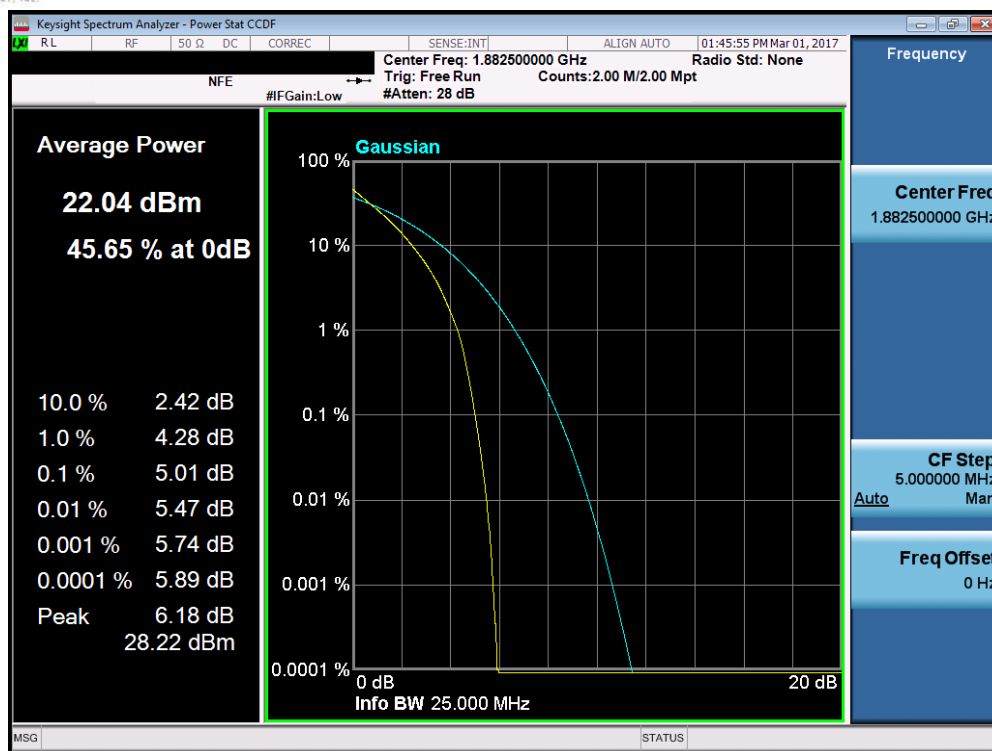
Plot 7-173. PAR Plot (Band 25 – 20.0MHz QPSK – RB Size 100)
