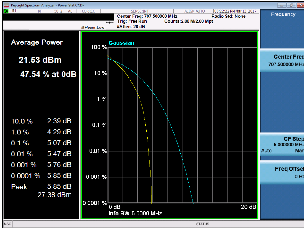
Plot 7-170. PAR Plot (Band 12 – 5.0MHz QPSK – RB Size 25)
