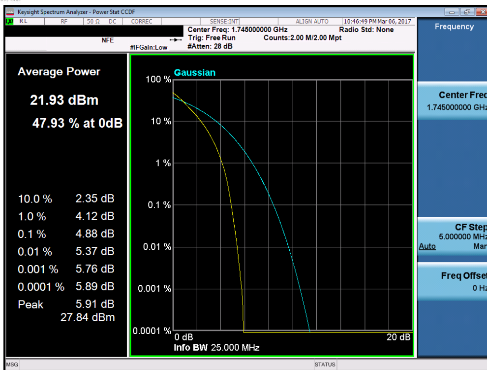
Plot 7-204. PAR Plot (Band 66 – 20.0MHz QPSK – RB Size 100)
