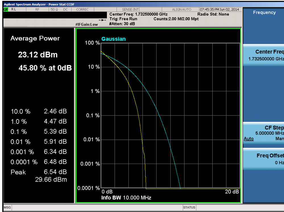
Plot 6-43. PAR Plot (Band 4 – 10.0MHz QPSK – RB Size 50)
