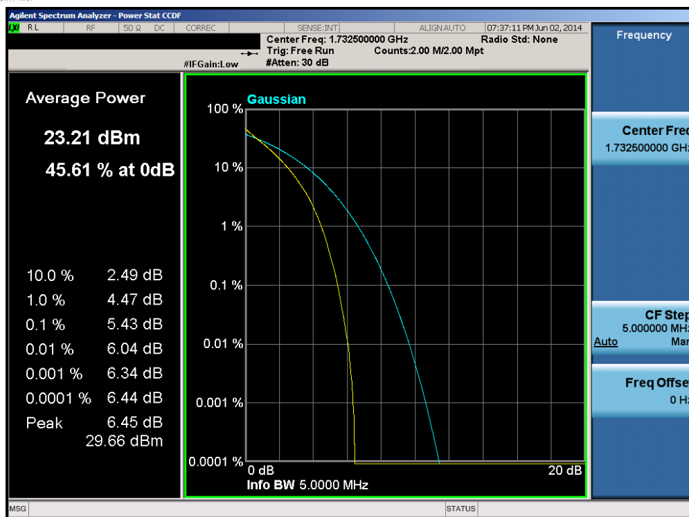
Plot 6-41. PAR Plot (Band 4 – 5.0MHz QPSK – RB Size 25)
