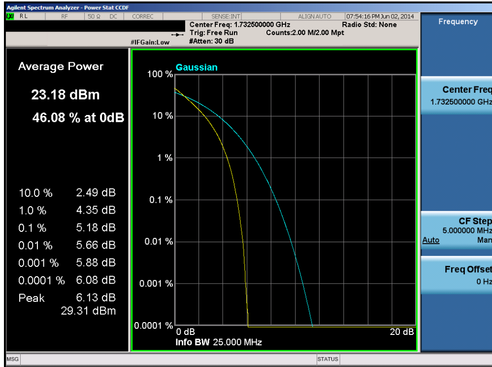
Plot 6-47. PAR Plot (Band 4 – 20.0MHz QPSK – RB Size 100)
