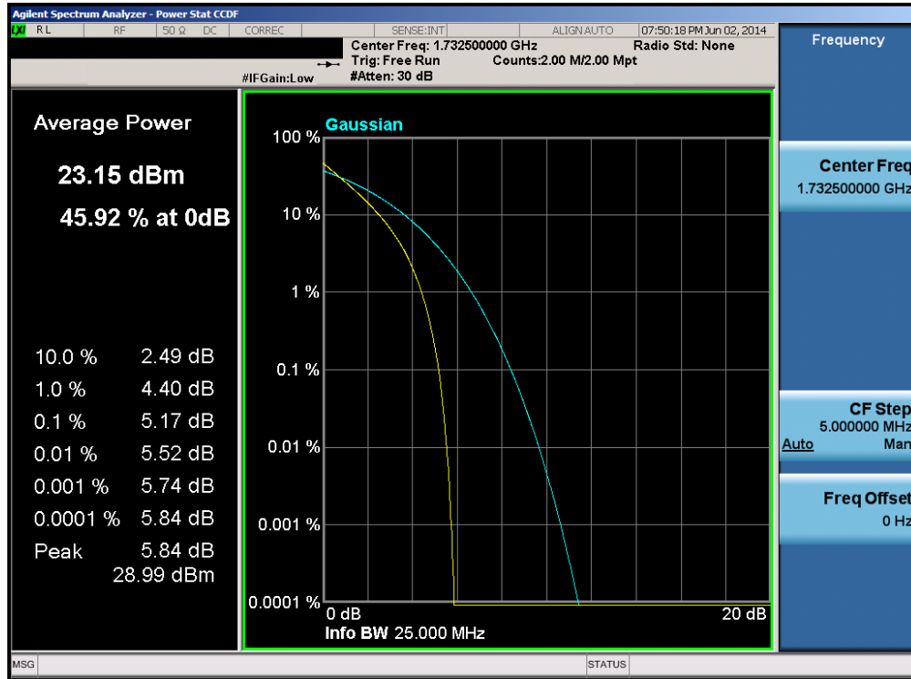
Plot 6-45. PAR Plot (Band 4 – 15.0MHz QPSK – RB Size 75)
