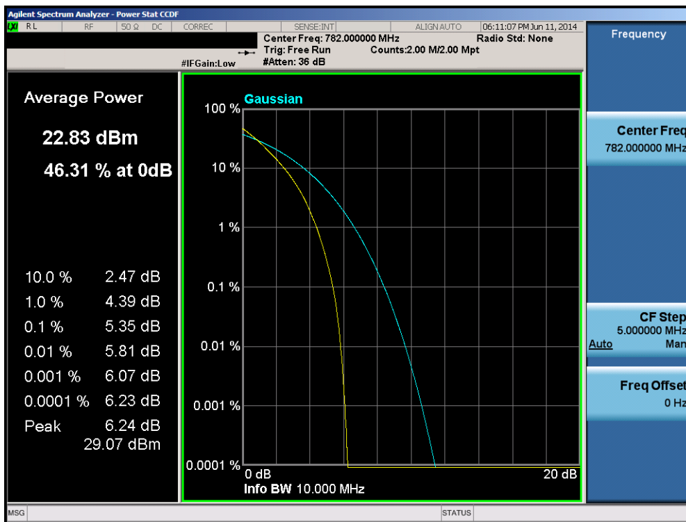
Plot 6-39. PAR Plot (Band 13 – 10.0MHz QPSK – RB Size 25)
