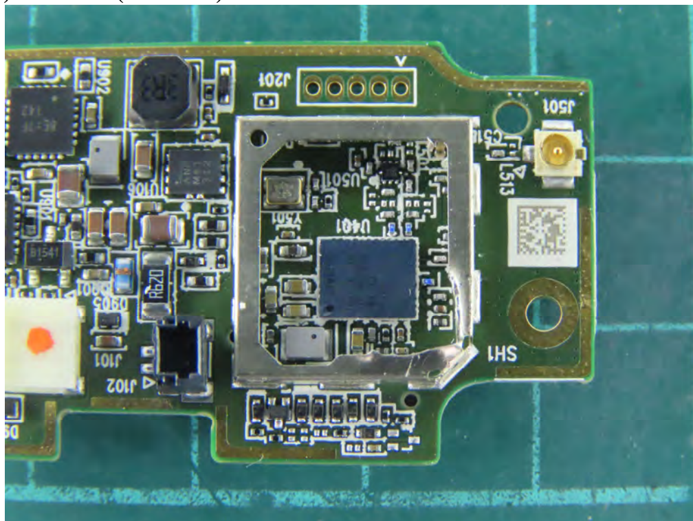
(43) EUT Photo (RF Module)
