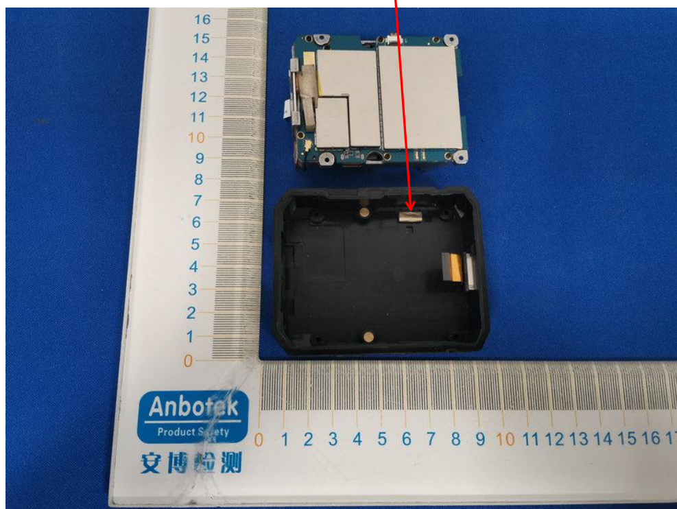
BT&WIFI ANT
