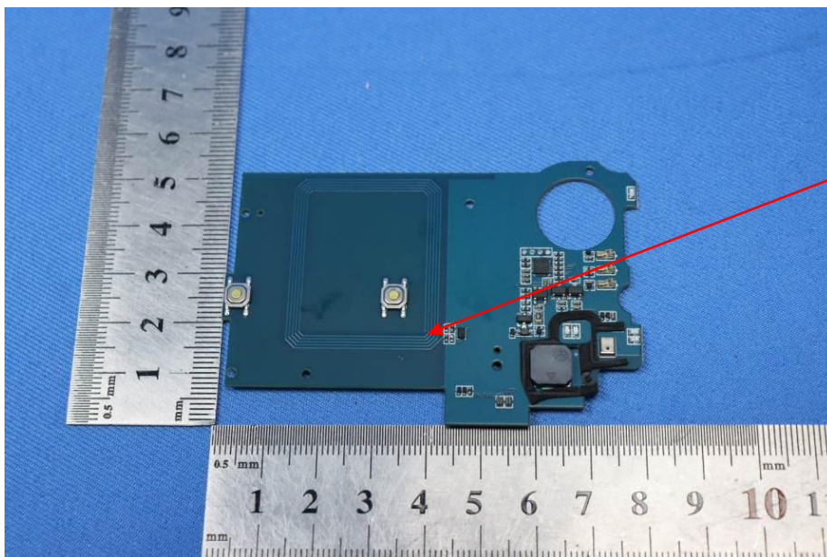
NFC(RX) antenna
