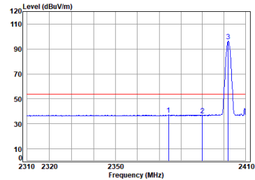
BLE_TX_CH_00_Horizontal-AVG
