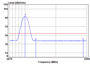
BLE_TX_CH_39_Horizontal-AVG
