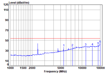
BLE_TX_CH_00_Horizontal-Avg
