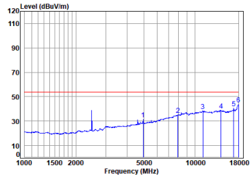
BLE_TX_CH_39_Vertical-Avg
