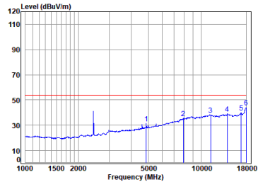
BLE_TX_CH_19_Vertical-Avg
