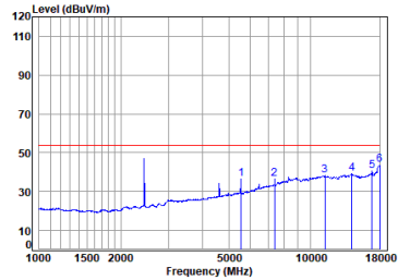
BLE_TX_CH_19_Horizontal-Avg
