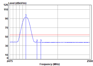
BLE_TX_CH_39_Vertical-AVG
