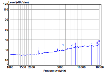
BLE_TX_CH_39_Horizontal-Avg
