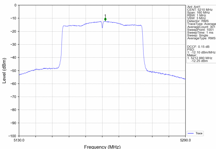
802.11ac(VHT80)_MCH_5210MHz_Ant1_NTNV
