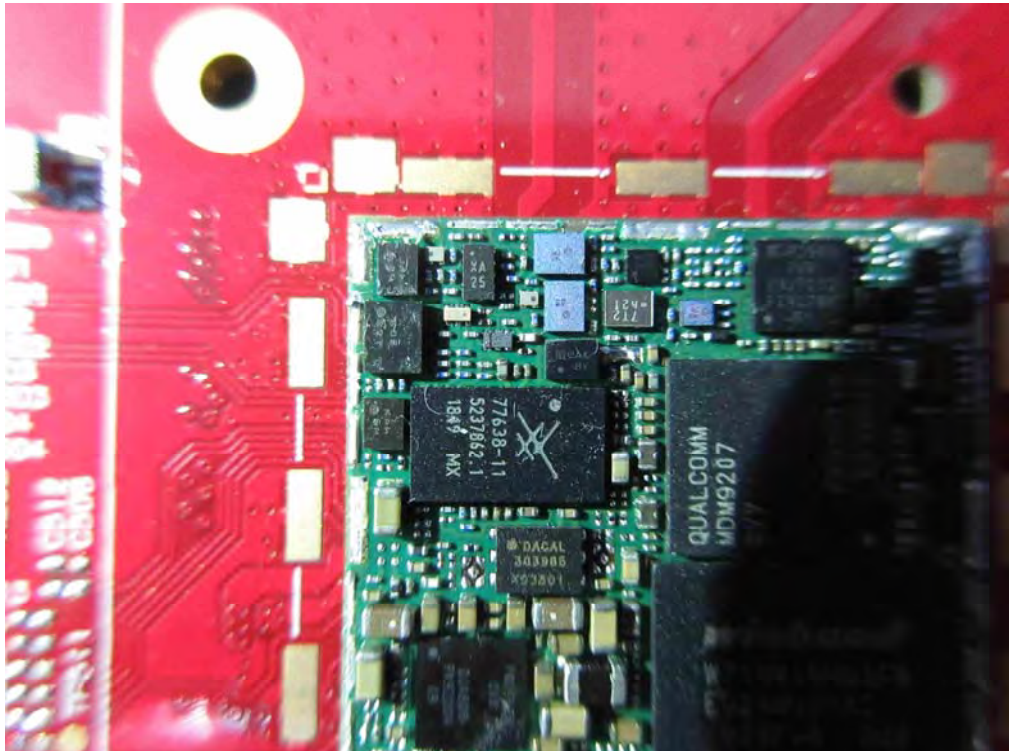
(9) EUT Photo
