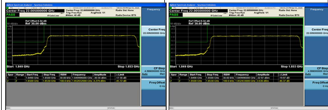
Band2-3MHz-QPSK-18615-15RB#0-PASS
