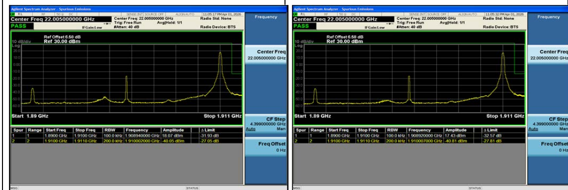
Band2-20MHz-QPSK-19100-1RB#99-PASS
