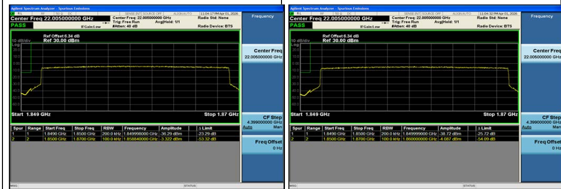
Band2-20MHz-QPSK-18700-100RB#0-PASS
