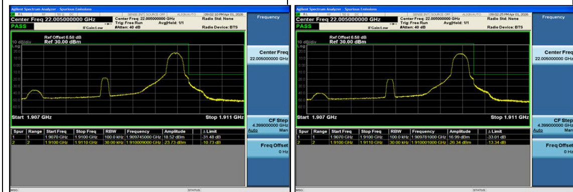
Band2-3MHz-QPSK-19185-1RB#14-PASS
