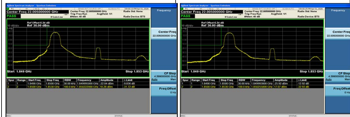
Band2-3MHz-QPSK-18615-1RB#0-PASS
