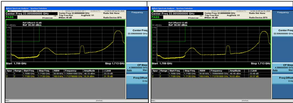
Band4-3MHz-QPSK-19965-1RB#14-PASS
