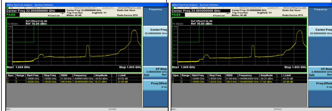
Band2-5MHz-QPSK-18625-1RB#24-PASS
