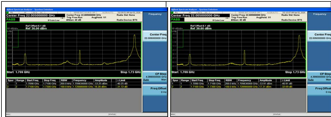
Band4-20MHz-QPSK-20050-1RB#99-PASS
