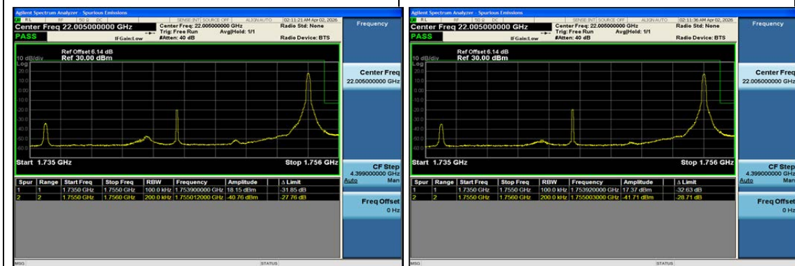
Band4-20MHz-QPSK-20300-1RB#99-PASS
