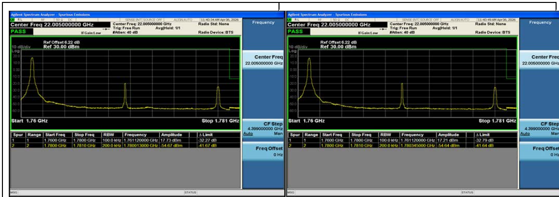
Band66-20MHz-QPSK-132572-1RB#0-PASS
