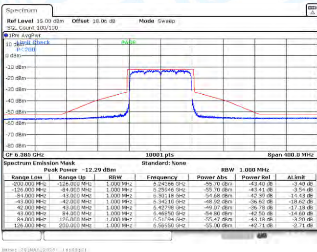
NTNV-11AX80SISO-Ant1-6385-PASS
