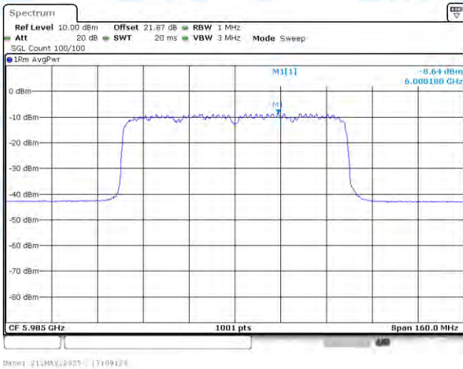
11AX80SISO-Ant1-5985-PASS
