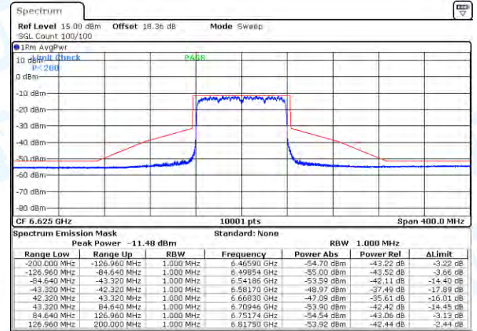
NTNV-11AX80SISO-Ant1-6625-PASS
