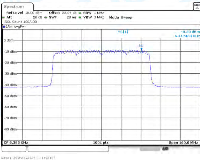
11AX80SISO-Ant1-6385-PASS
