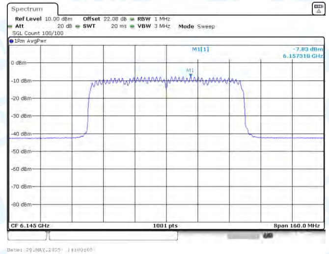
11AX80SISO-Ant1-6145-PASS
