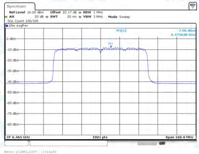
11AX80SISO-Ant1-6465-PASS
