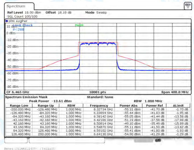
NTNV-11AX80SISO-Ant1-6465-PASS
