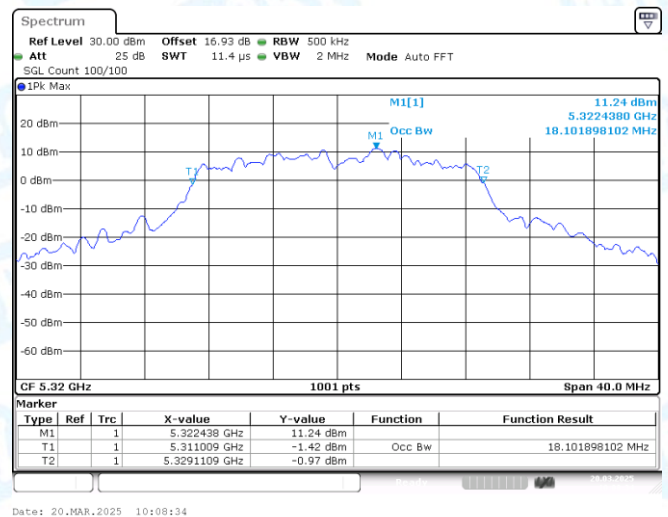
11N20MIMO-Ant1-5320
