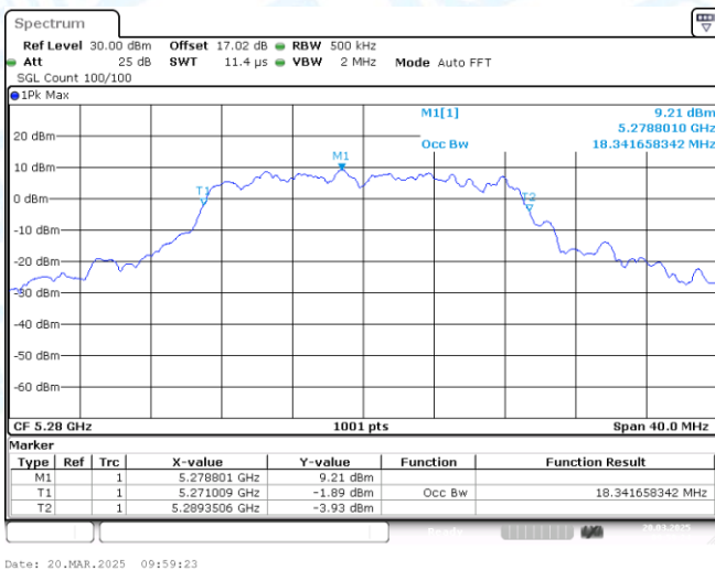
11N20MIMO-Ant2-5280
