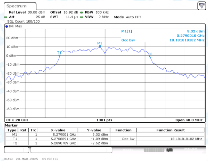
11N20MIMO-Ant1-5280
