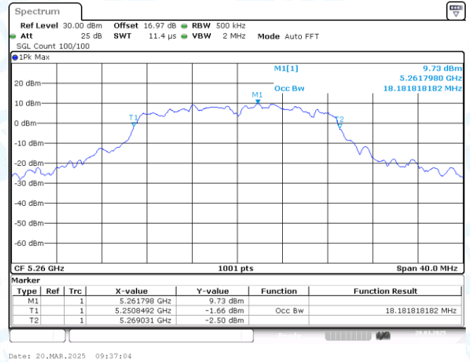
11N20MIMO-Ant1-5260
