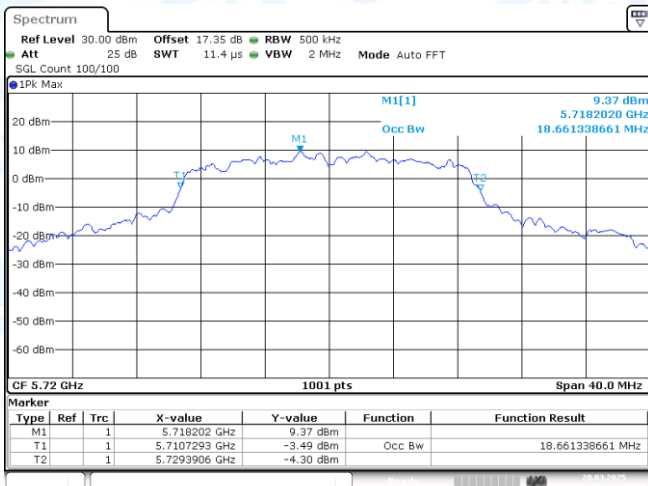
11N20MIMO-Ant2-5700
