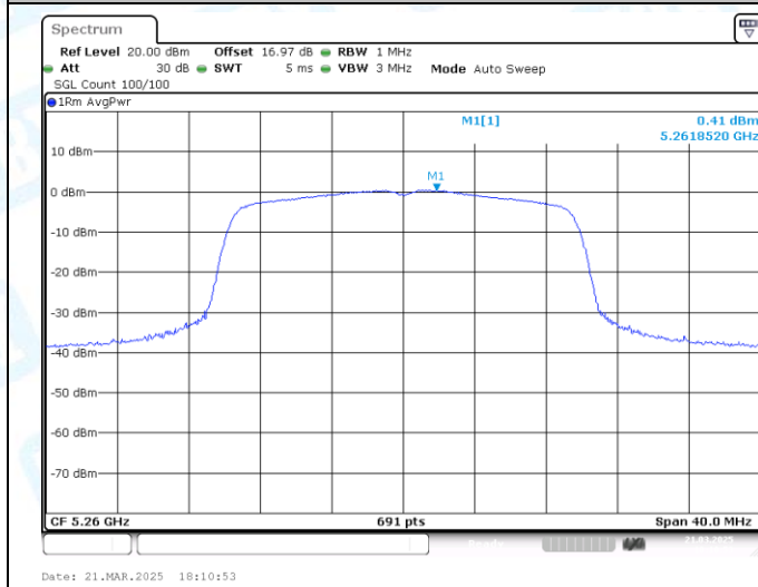
11AX20MIMO-Ant1-5260-PASS
