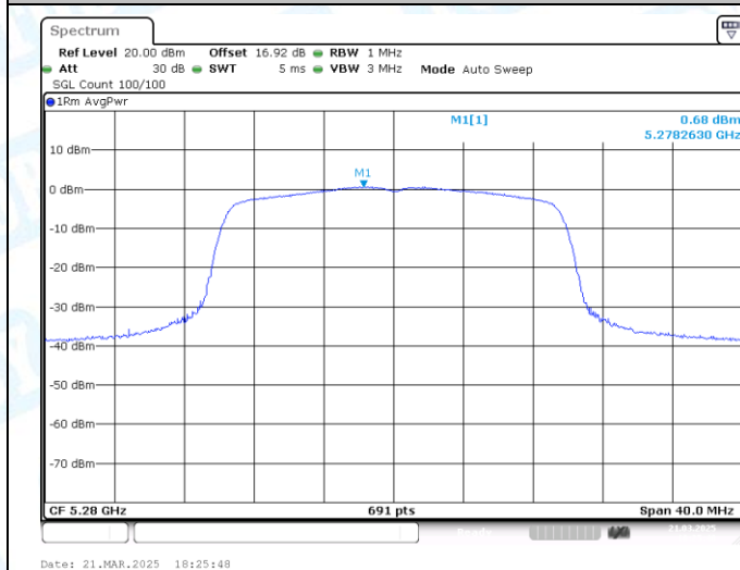
11AX20MIMO-Ant1-5280-PASS
