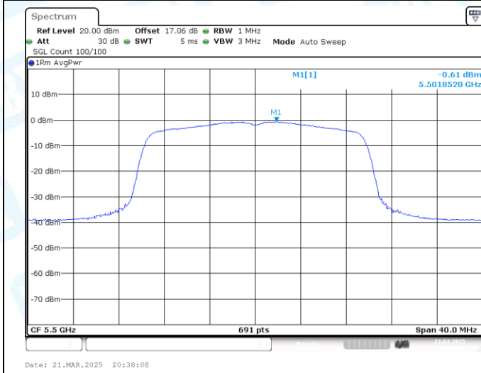
11AX20MIMO-Ant1-5500-PASS
