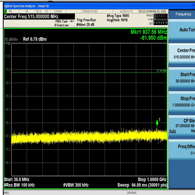
BLE_2M-Ant1-2440-30~1000-PASS
