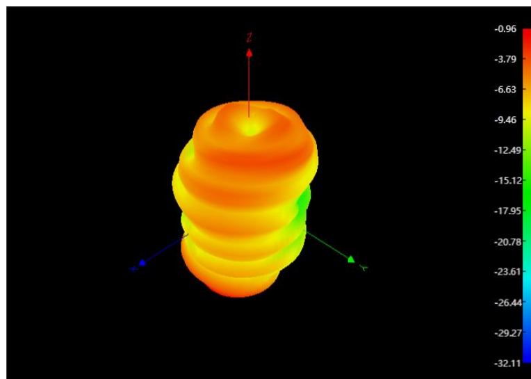
2500MHz 3D
