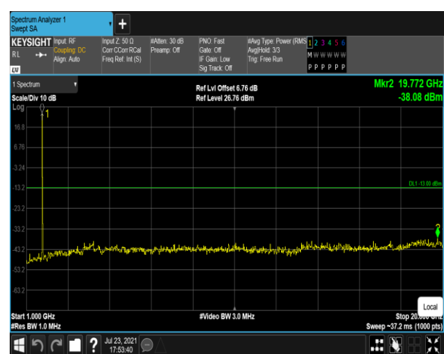
Band4-20MHz-QPSK-20050-1RB#0-Range2:1000~20000MHz
