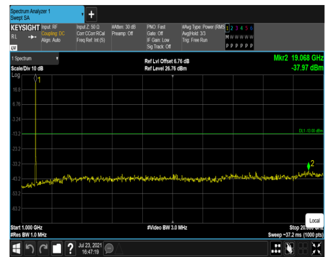
Band2-20MHz-16QAM-18900-1RB#0-Range2:1000~2 0000MHz
