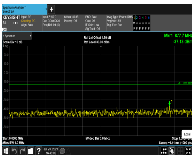
Band2-20MHz-16QAM-19100-1RB#0-Range1:30~ 1000MHz
