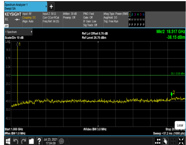
Band4-1.4MHz-QPSK-19957-1RB#0-Range2:1000~2 0000MHz
