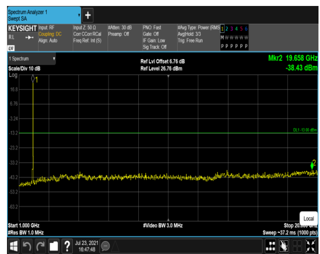
Band2-20MHz-QPSK-19100-1RB#0-Range2:1000~20 000MHz
