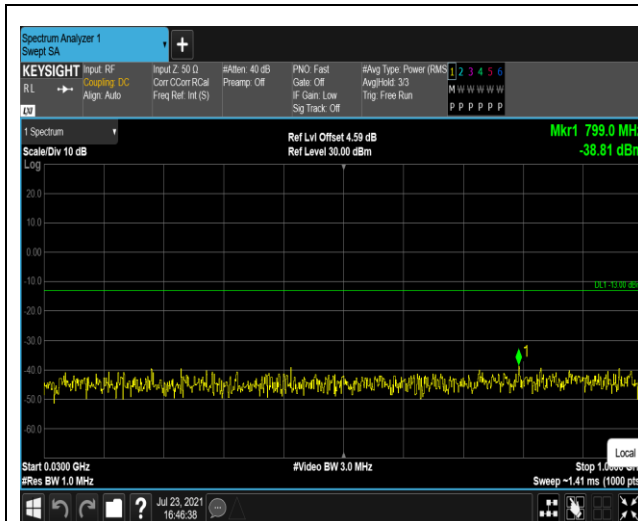
Band2-20MHz-QPSK-18900-1RB#0-Range1:30~1 000MHz
