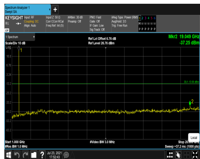
Band4-20MHz-QPSK-20050-1RB#0-Range2:1000~20000MHz
