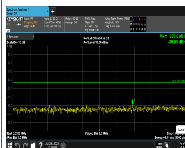
Band2-20MHz-QPSK-19100-1RB#0-Range1:30~1 000MHz
