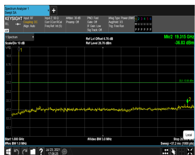
Band4-1.4MHz-QPSK-20175-1RB#0-Range2:1000~2 0000MHz
