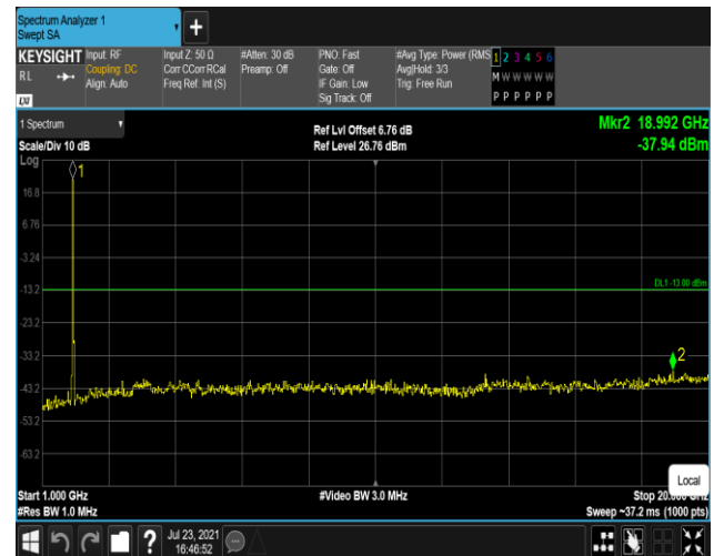
Band2-20MHz-QPSK-18900-1RB#0-Range2:1000~20 000MHz
