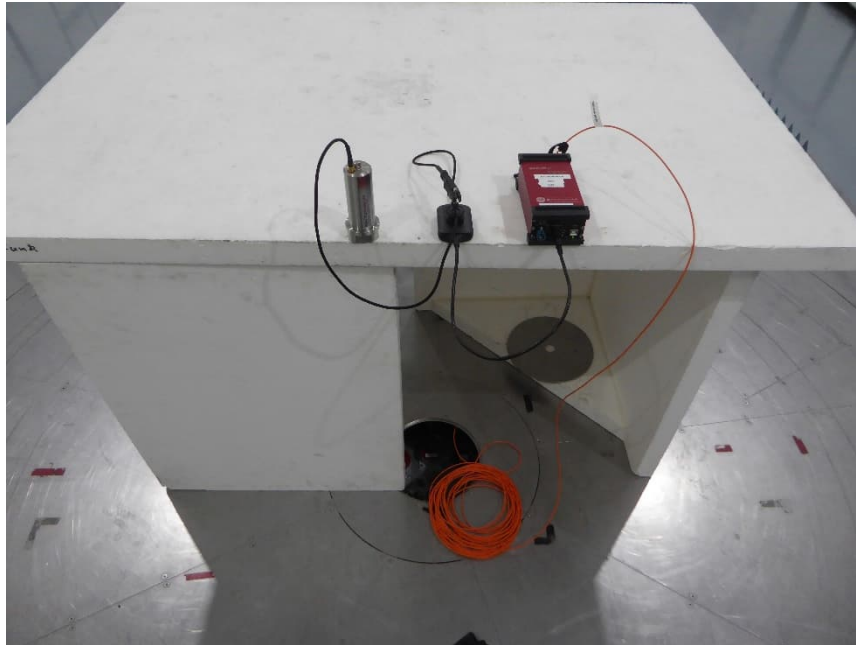
EUT setup
