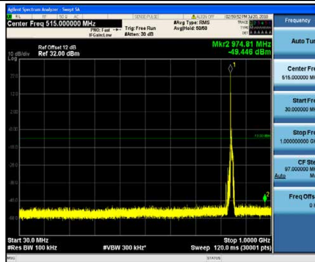
Band5_10MHz_QPSK_20635_1RB#0
