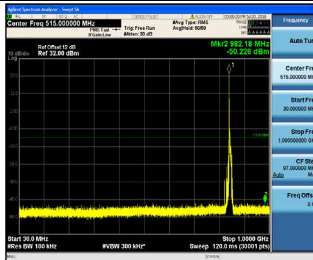
Band5_10MHz_16QAM_20635_1RB#0
