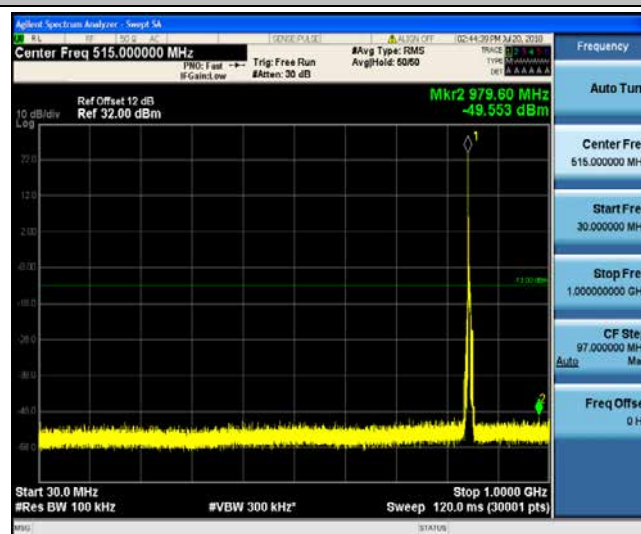
Band5_5MHz_16QAM_20635_1RB#0
