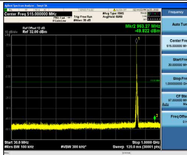
Band5_5MHz_QPSK_20635_1RB#0
