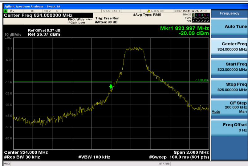
Band5-3MHz-QPSK-20415-1RB#0
