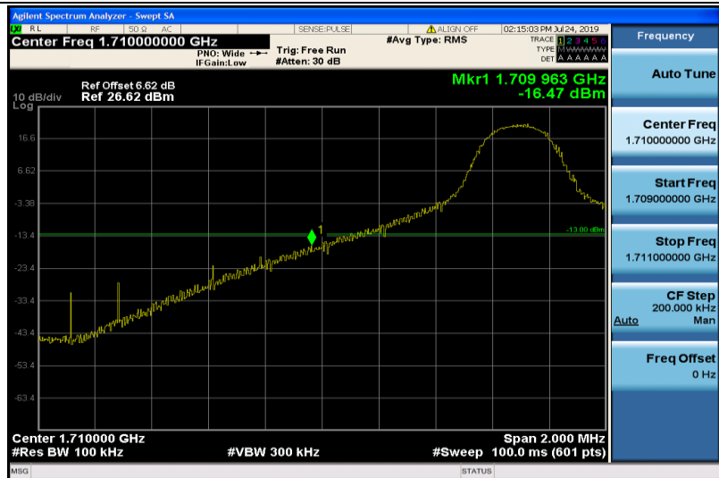
Band4-10MHz-QPSK-20000-1RB#0
