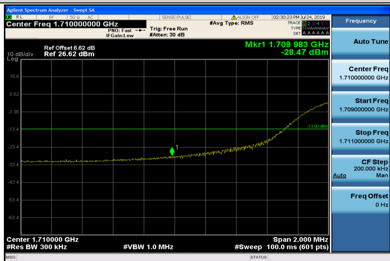
Band4-20MHz-QPSK-20050-100RB#0
