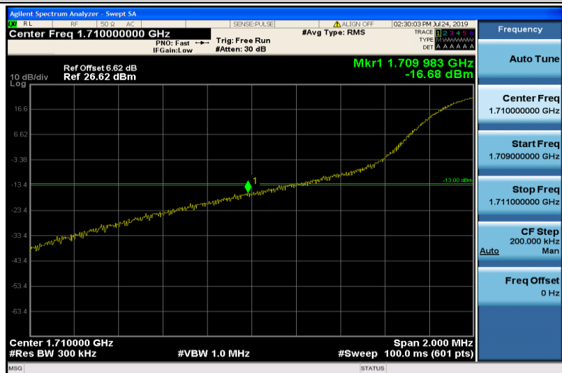
Band4-20MHz-QPSK-20050-1RB#0
