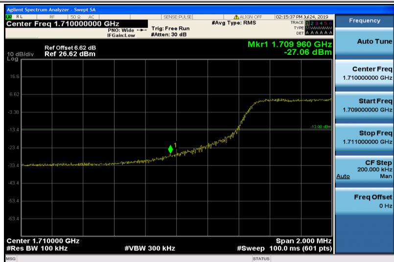
Band4-10MHz-QPSK-20000-50RB#0
