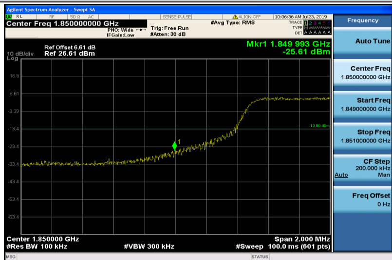
Band2-10MHz-QPSK-18650-50RB#0
