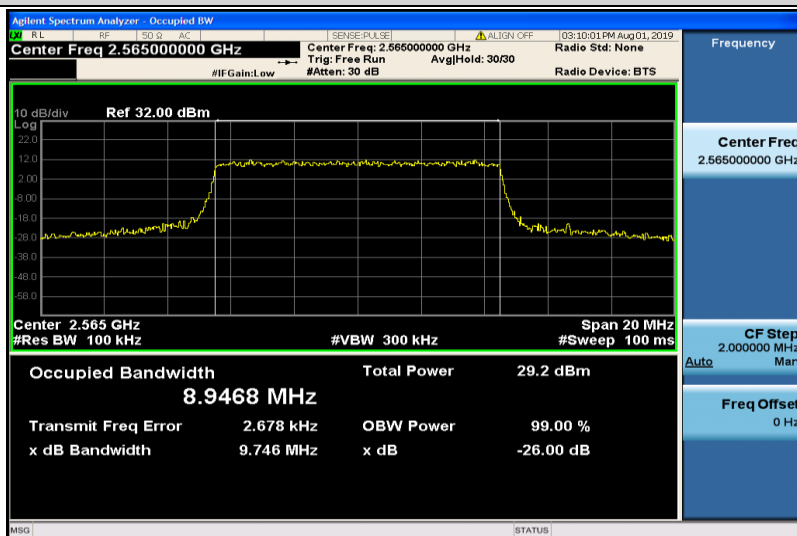
Band7-10MHz-QPSK-21400-50RB#0-8.9468
