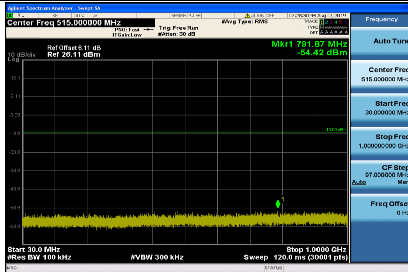
Band2-3MHz-QPSK-18615-1RB#0-30~1000MHz
