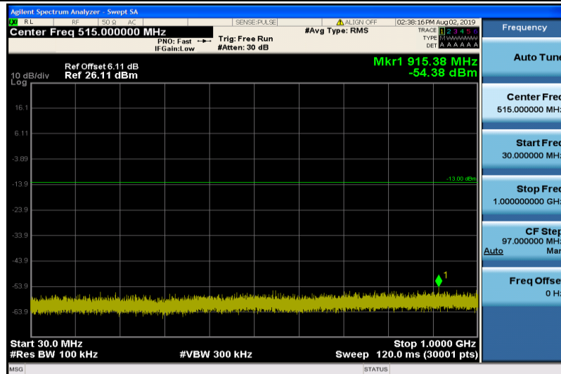
Band2-5MHz-QPSK-19175-1RB#0-30~1000MHz
