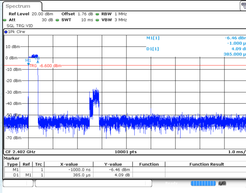
DH1
