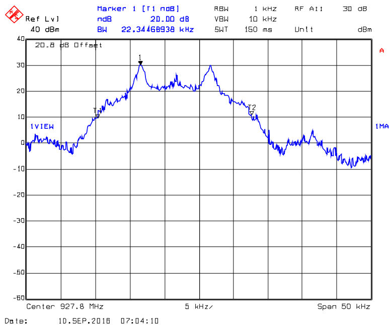
Plot 5.3.4.12. 20 dB Bandwidth, 927.8 MHz, DSSS1, 10 kbps-Right Antenna
