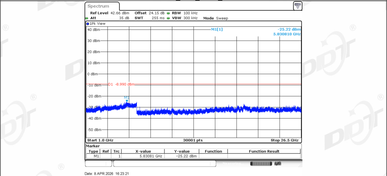
LORA DTS SF12_Ant1_923.3_0~Reference
