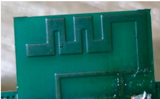
wireless TX天线
