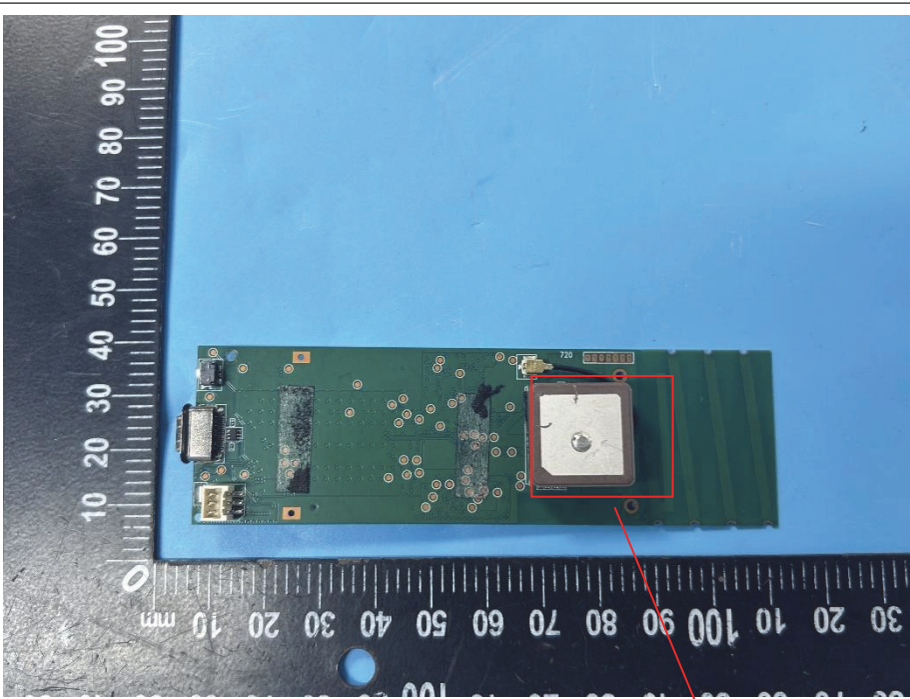
GPS Ant(RX).
