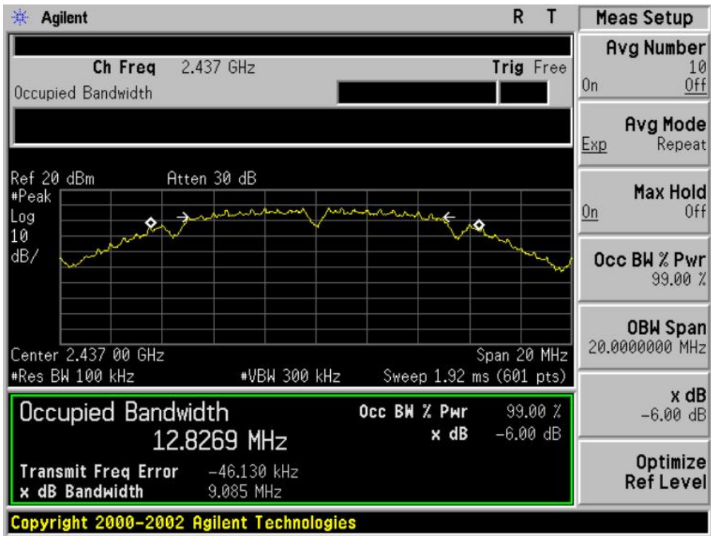
802.11b 2437MHz
