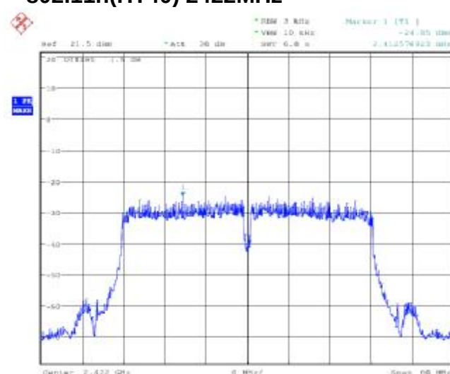
802.11n(HT40) 2422MHz
