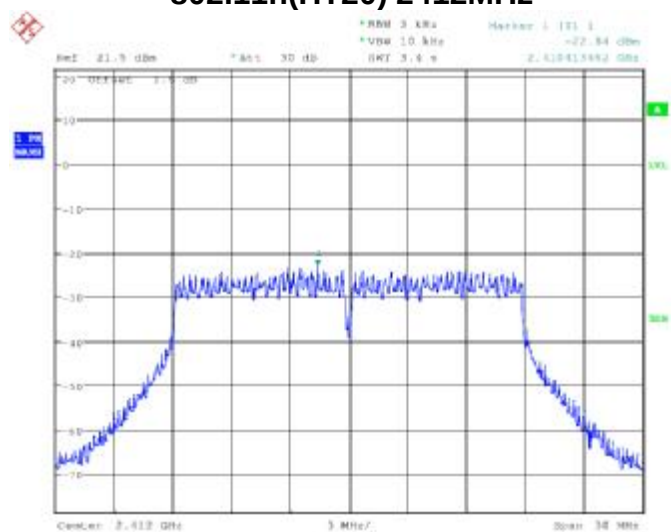
802.11n(HT20) 2412MHz
