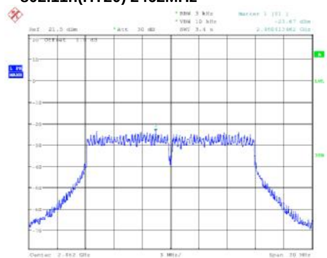
802.11n(HT20) 2462MHz
