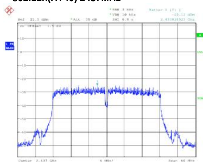
802.11n(HT40) 2437MHz
