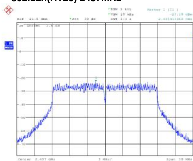
802.11n(HT20) 2437MHz
