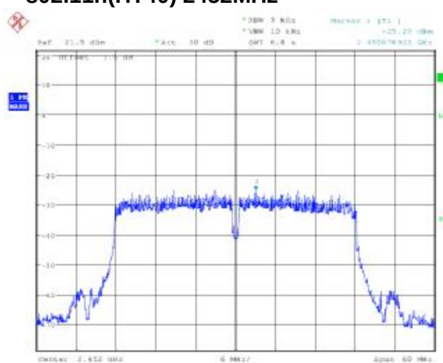
802.11n(HT40) 2452MHz
