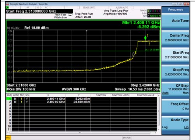
802.11n HT20-2412
