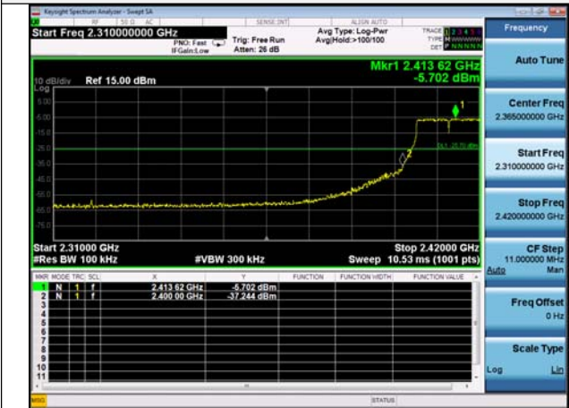
802.11g-2412
