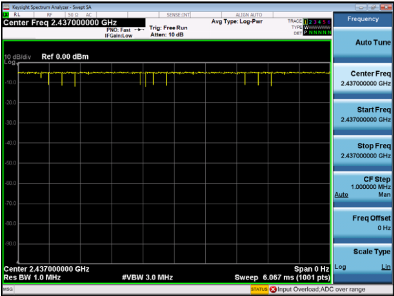
802.11b-2437MHz
