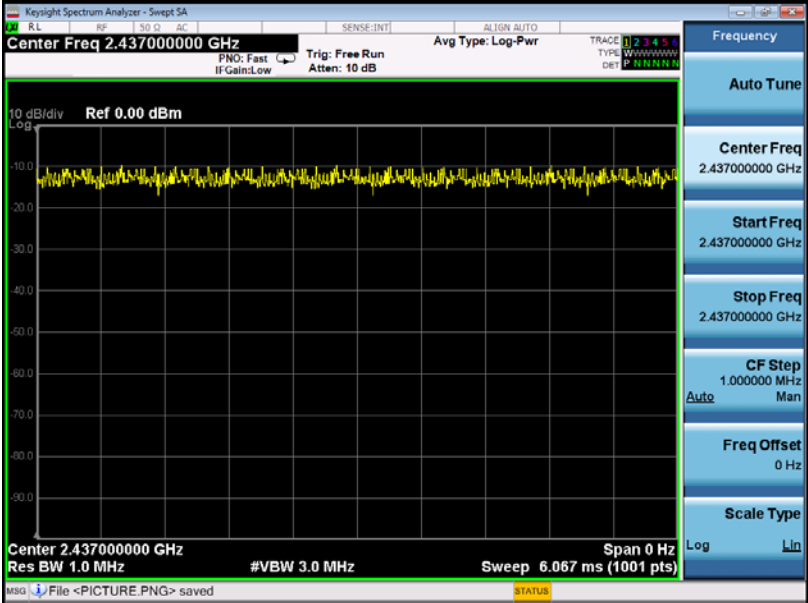
802.11n20-2437MHz
