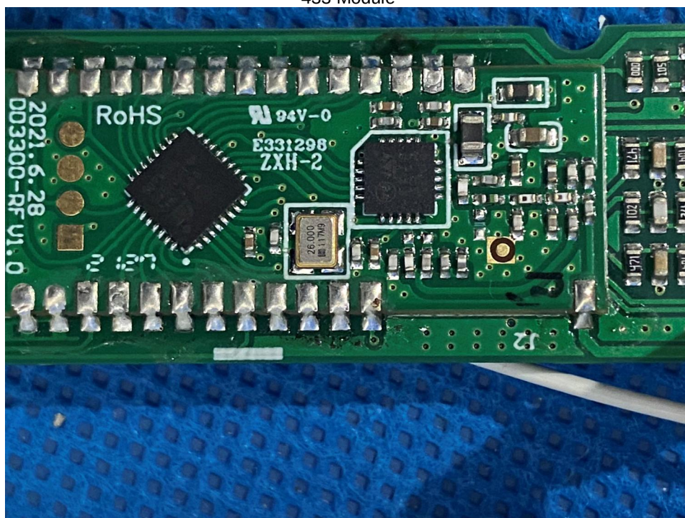
433 Module
