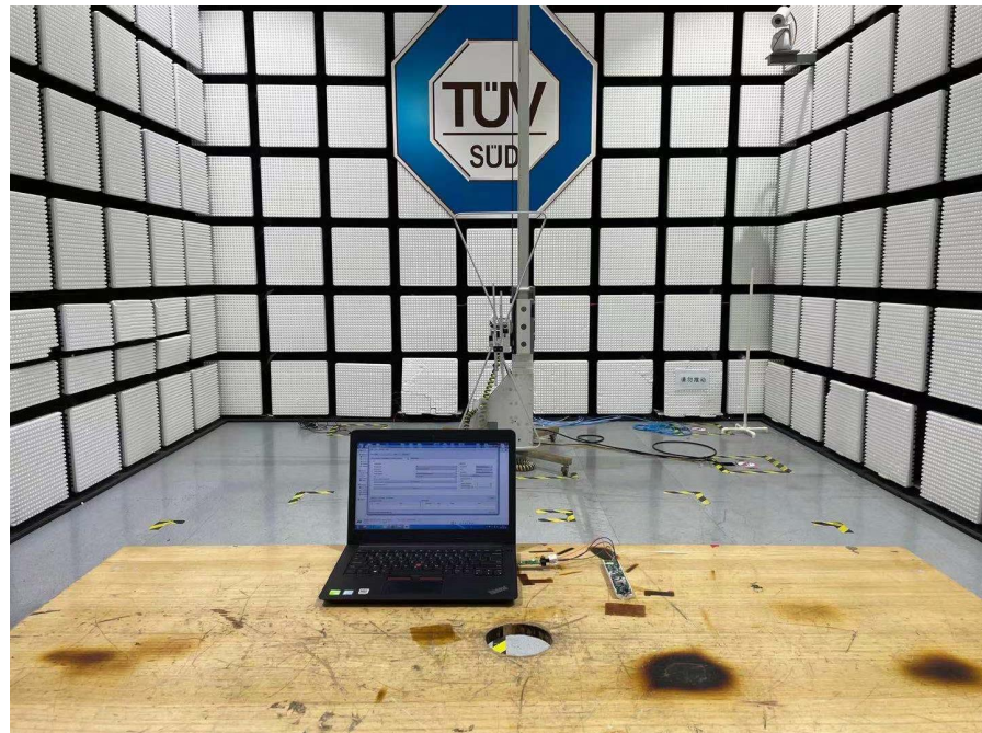
30MHz ~ 1GHz
