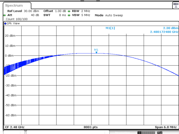
BLE_Ant1_2480
