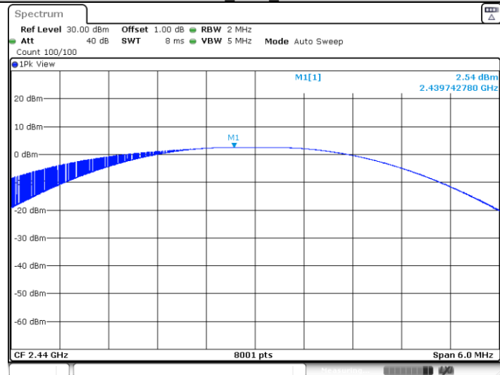
BLE_Ant1_2440
