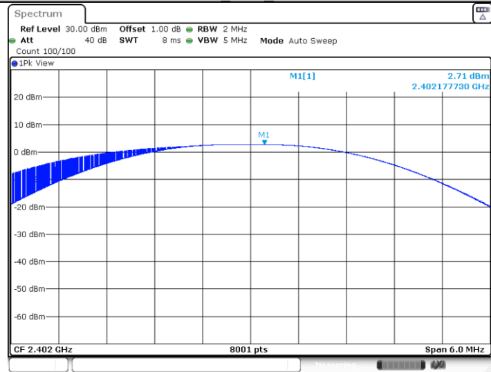
BLE_Ant1_2402
