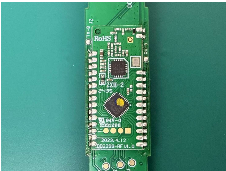
Internal: 433 Module
