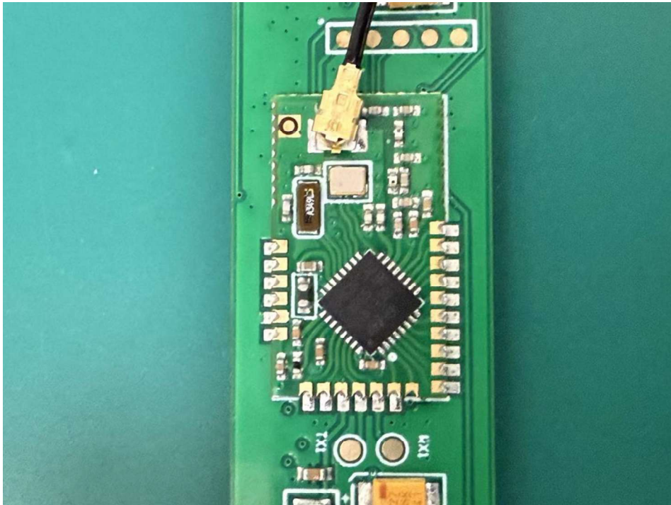
Internal: BLE Module
